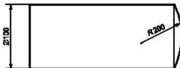
Рисунок В.4 — Испытательный груз
