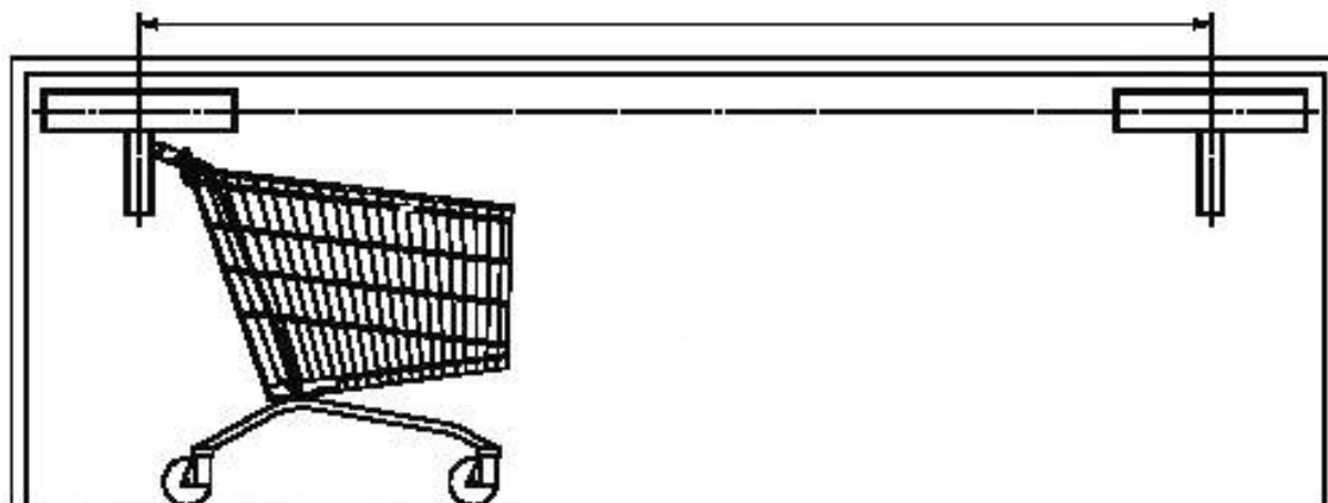
Рисунок В.7 — Схема испытания на долговечность
