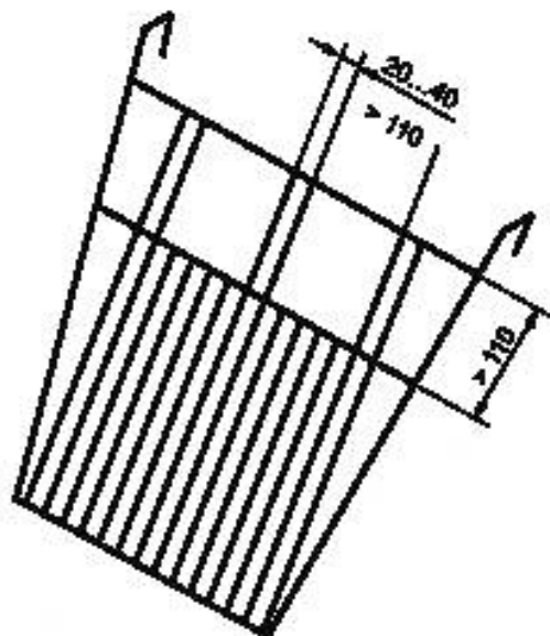
Рисунок Б.3 — Проходные отверстия для ног
