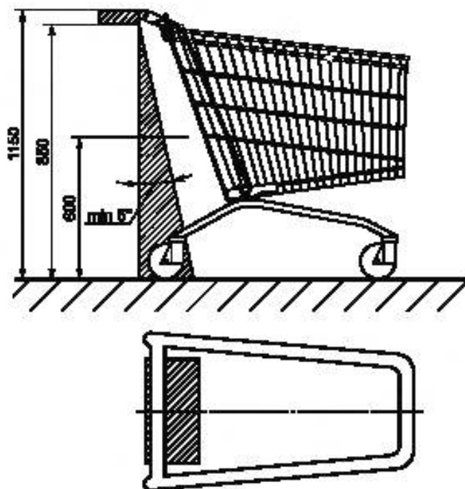
Рисунок 4 — Пространство для ног
