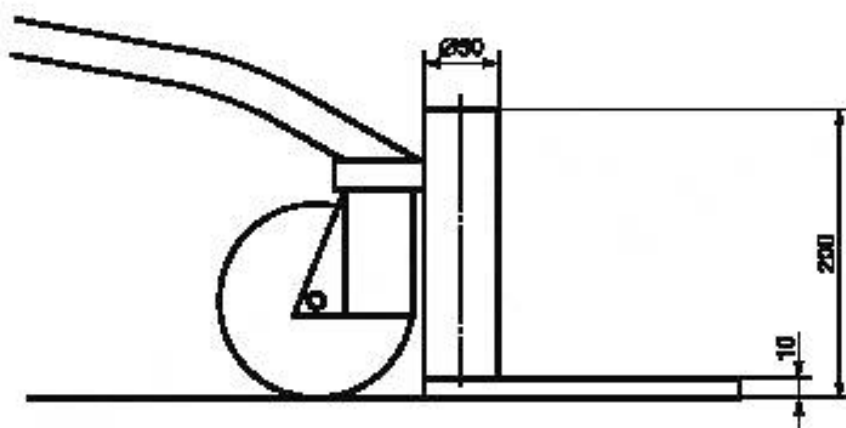
Рисунок В.9 — Испытательное оборудование
