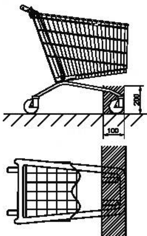
Рисунок В.10 — Пространство для испытания
