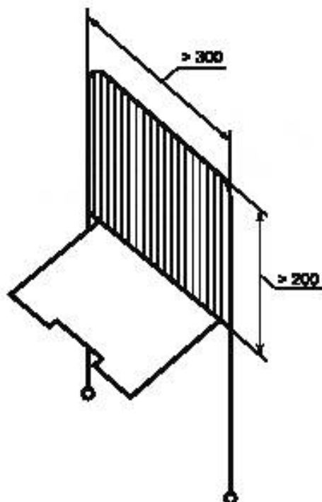
Рисунок Б.2 — Откидная стенка
