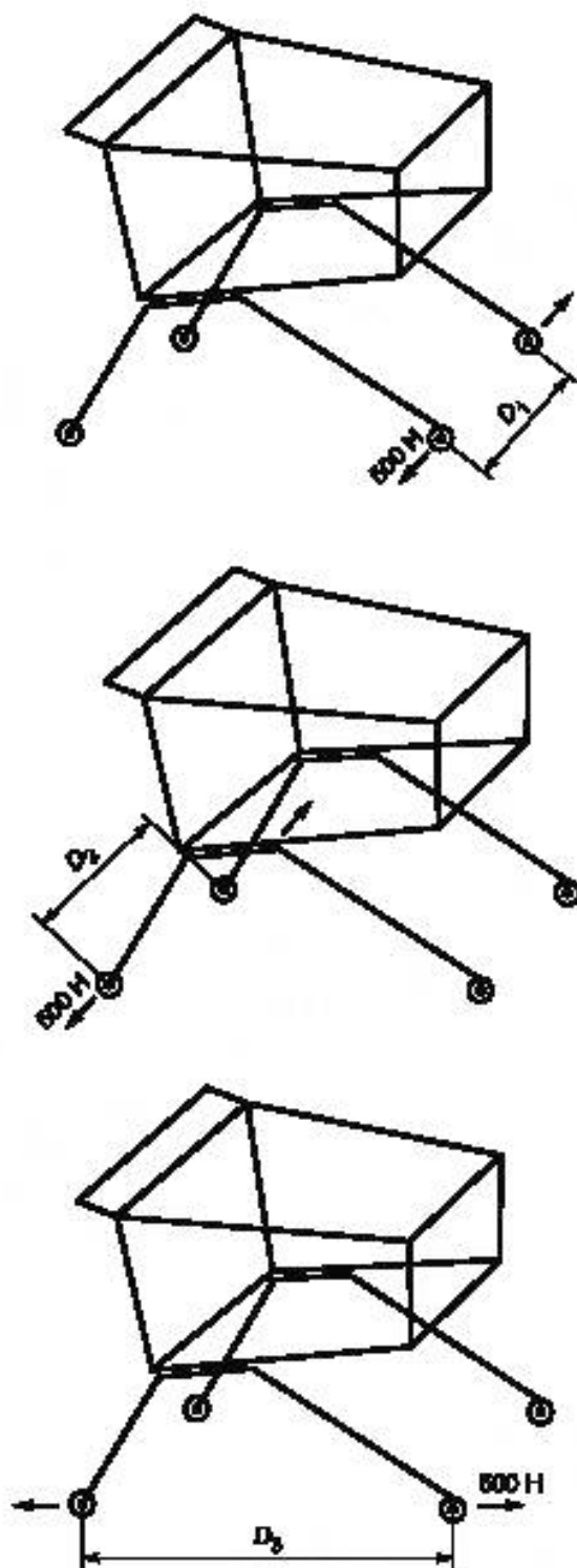
Рисунок В.6 — Схемы испытания рамы на прочность
