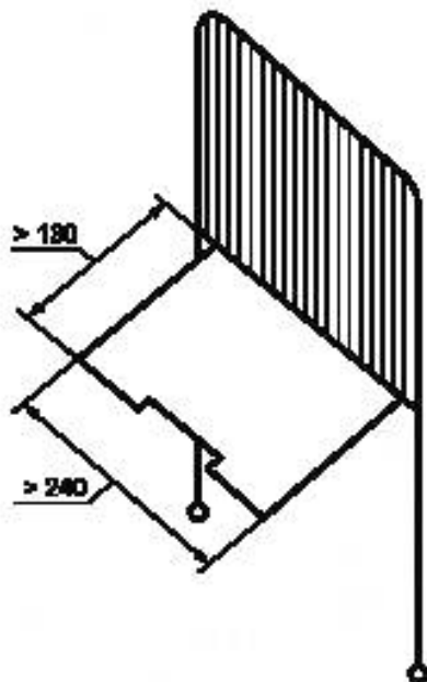
Рисунок Б.1 — Рабочее положение опорной поверхности
