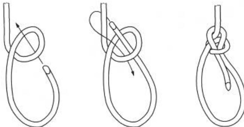
Рисунок 3 — Узел булинь
