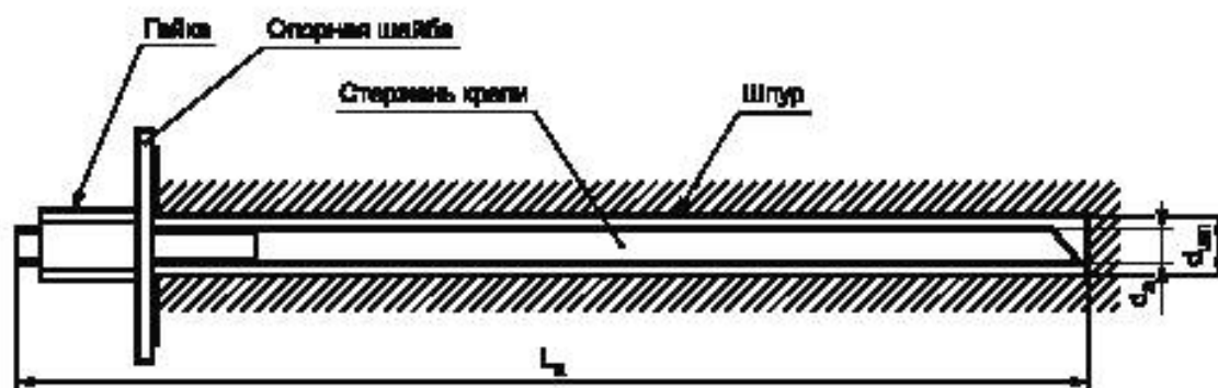
Рисунок 1 — Принципиальная схема крепи анкерной
