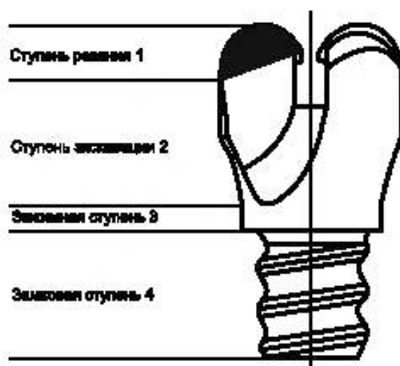
Рисунок 2 — Конструкция бурового резца
