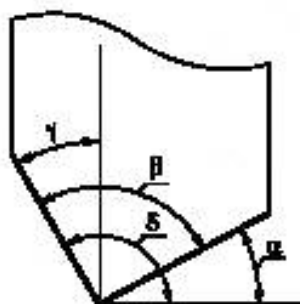
Рисунок 1 — Конструктивные углы
