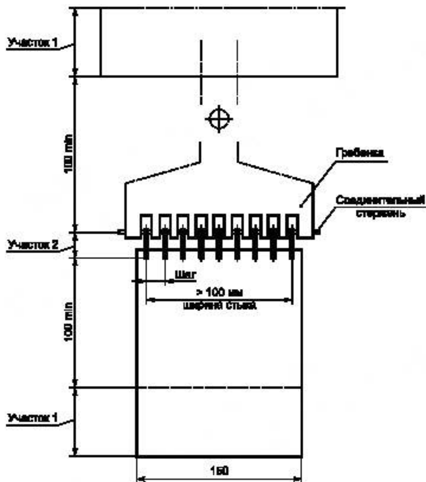
Рисунок 3 — Образец разъемного механического соединения с использованием гребенки
