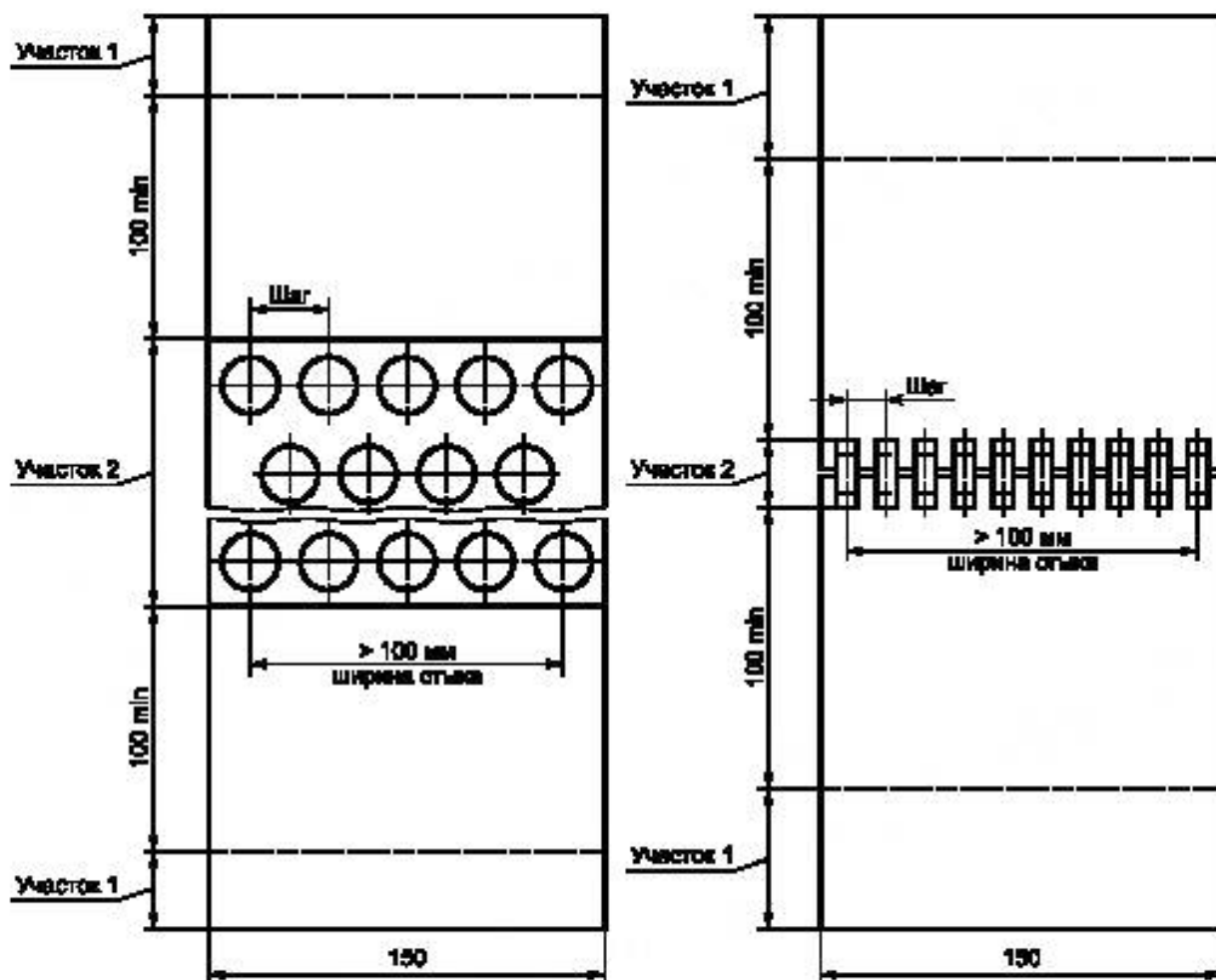
Рисунок 1 — Образцы неразъемного механического соединения
