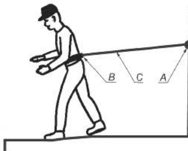
А — анкерная точка; В — привязь; С — строп
