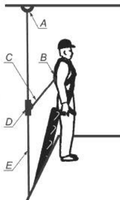
А — анкерная точка; В — страховочная привязь; С — строп; D — устройство ползункового типа; E — гибкая анкерная линия
