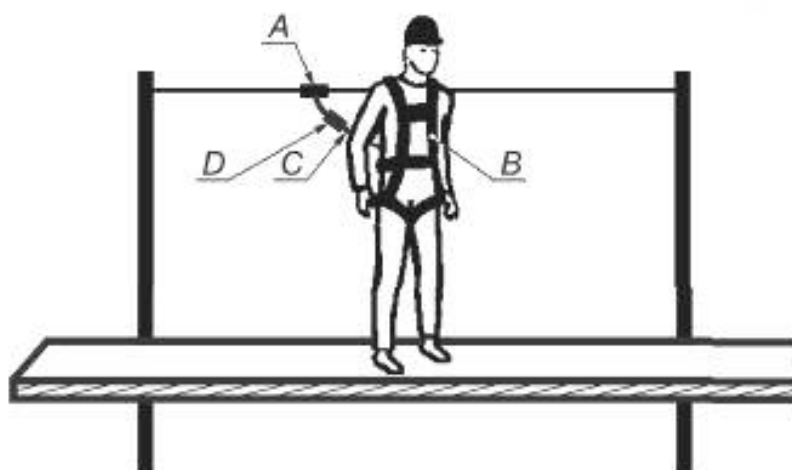
Рисунок 5 — Пример страховочной системы со стропом и амортизатором
