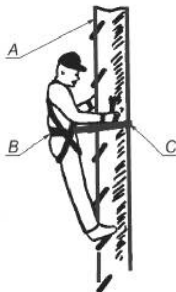
A — крепление; B — привязь; C — строп для системы позиционирования (применяется для работ на столбах)
