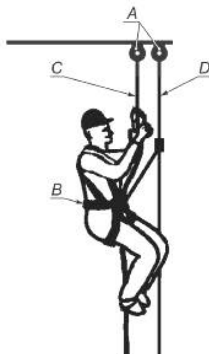
А — анкерная точка; В — привязь; С — рабочий канат; D — страховочный канат
