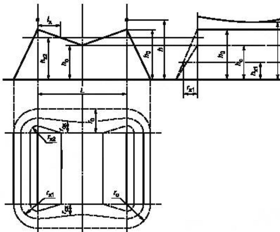
Рисунок А.5 — Зона защиты двойного тросового молниеотвода
