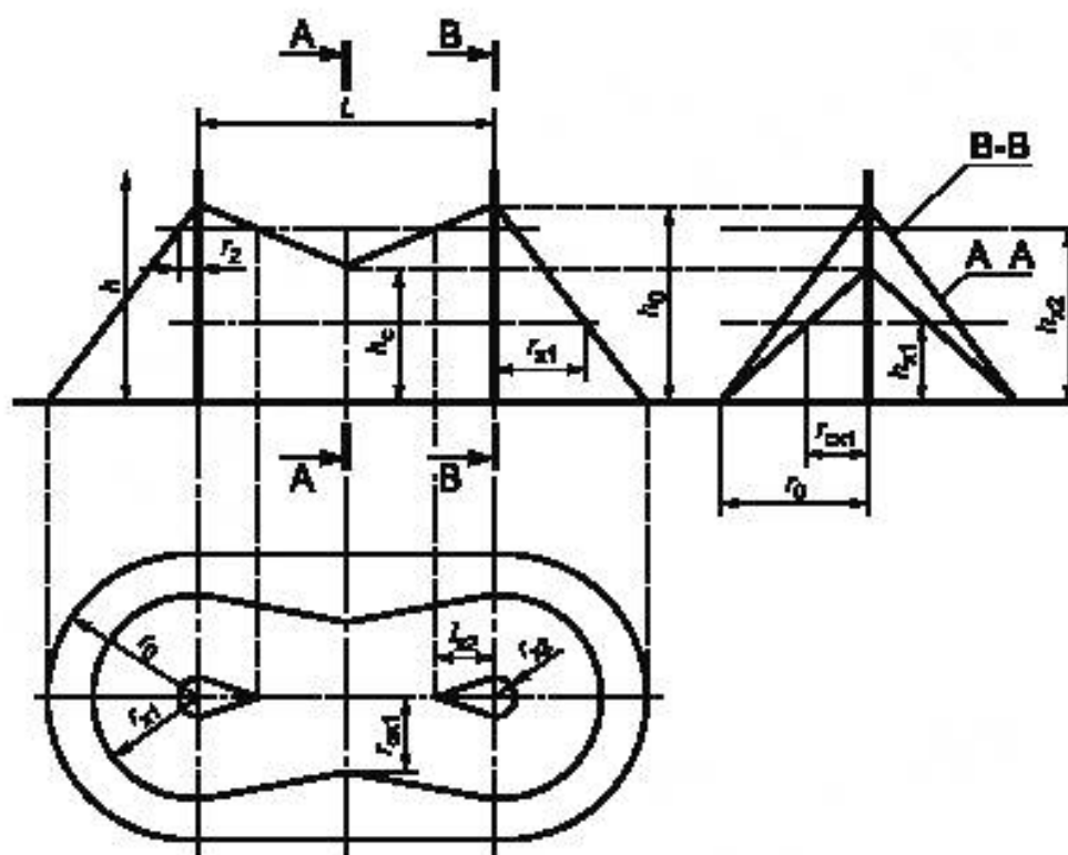
Рисунок А.3 — Зона защиты двойного стержневого молниеотвода
