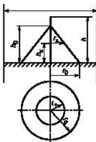
Рисунок А.1 — Зона защиты одиночного стержневого молниеотвода
