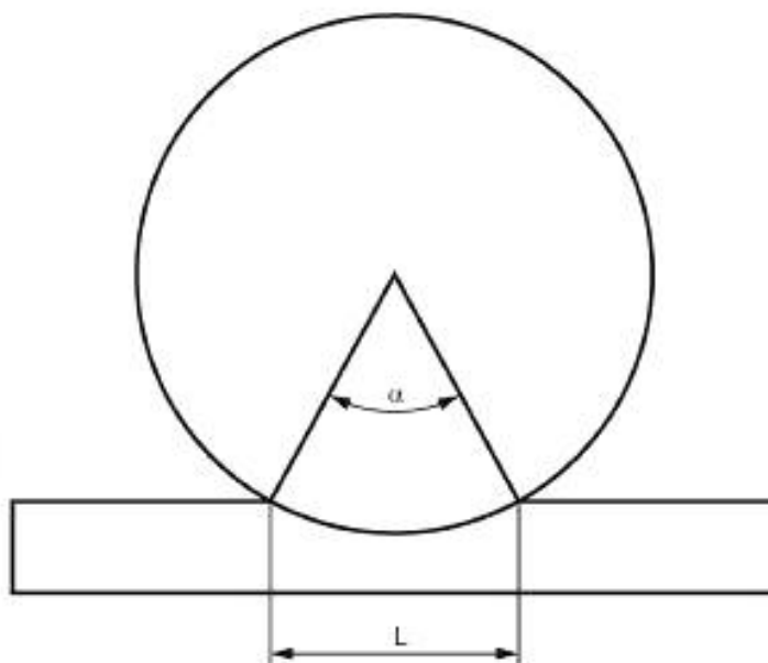
Рисунок А.2 — Определение угла и хорды
