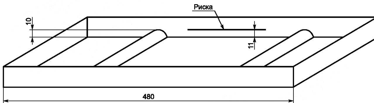
Рисунок 10 — Емкость для выдержки образцов в воде
