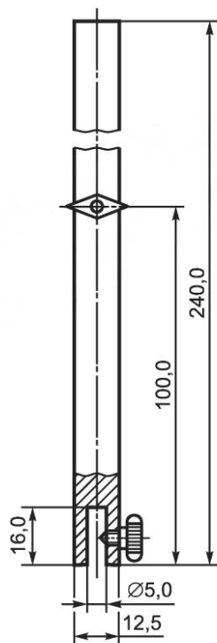
б) Подвижный стержень, материал — алюминиевый сплав
