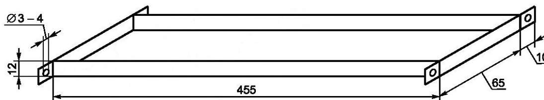
в) Рама для крепления образца
