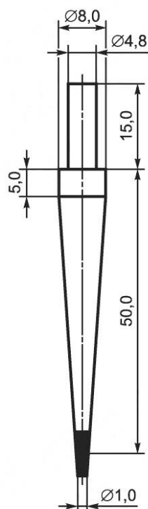
а) Съемный конус, материал — сталь
