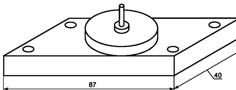
Рисунок 9 — Держатель шлифующей шкурки
