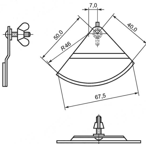
Рисунок 3 — Пластика-фиксатор подвижного стержня с конусом
