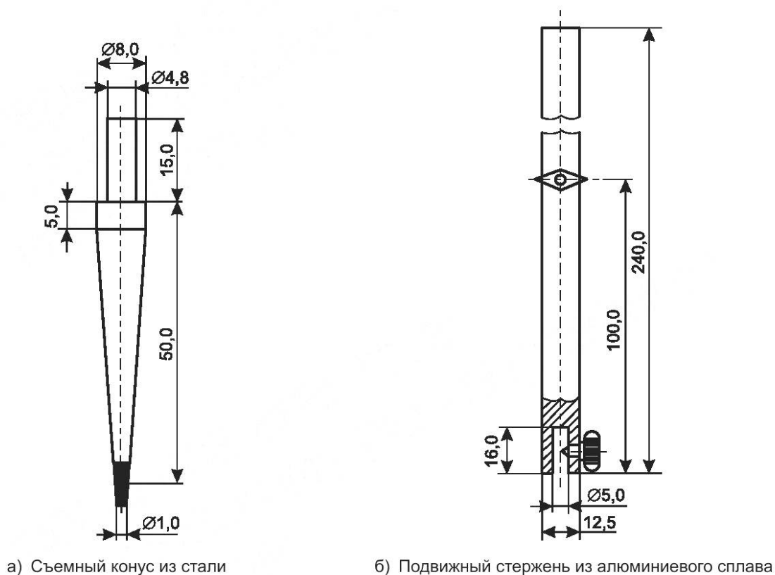
Рисунок 2 — Подвижная часть прибора Вика
