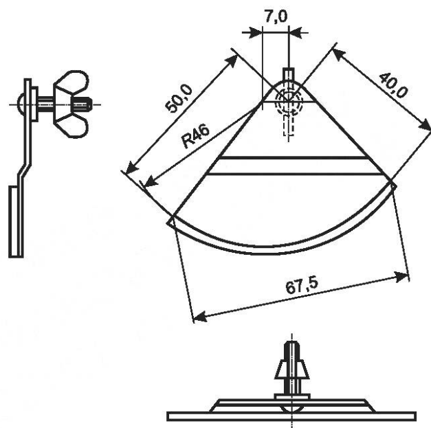
Рисунок 3 — Пластика-фиксатор подвижного стержня с конусом
