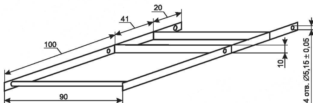
г) Каретка с ручкой
