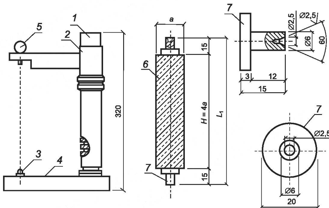
1 — стойка; 2 — кронштейн; 3 — конусообразный выступ; 4 — нижняя опора; 5 — индикатор часового типа; 6 — образец; 7 — репер; а — размер стороны поперечного сечения образца; H — высота образца; L 1 — база измерений
