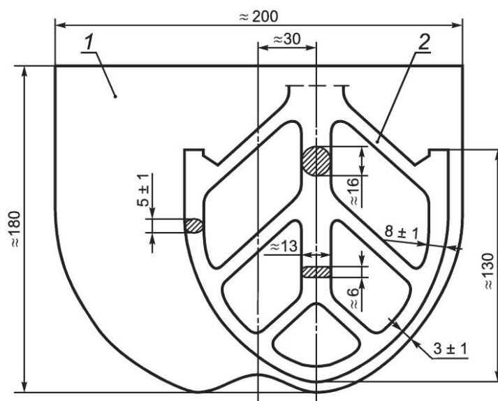
1 — чаша; 2 — лопасть
