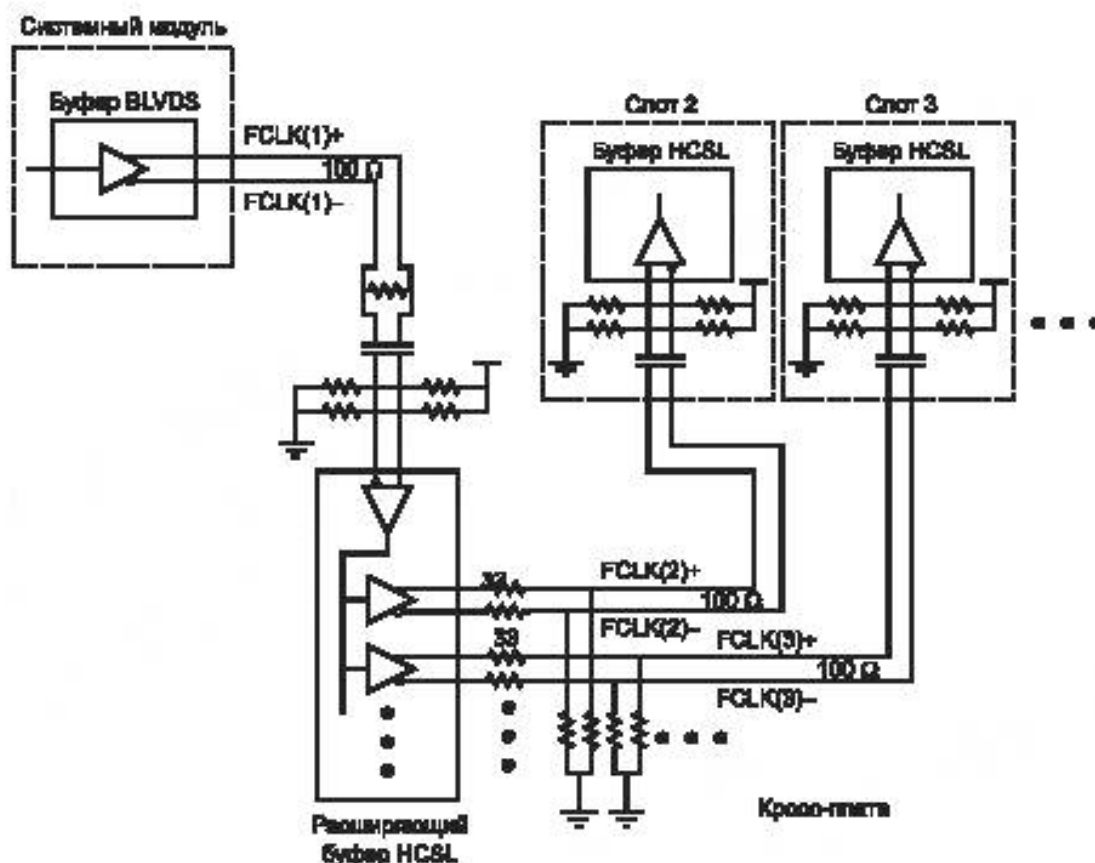
Рисунок 6.7 — Типичная реализация сигнала FCLK
