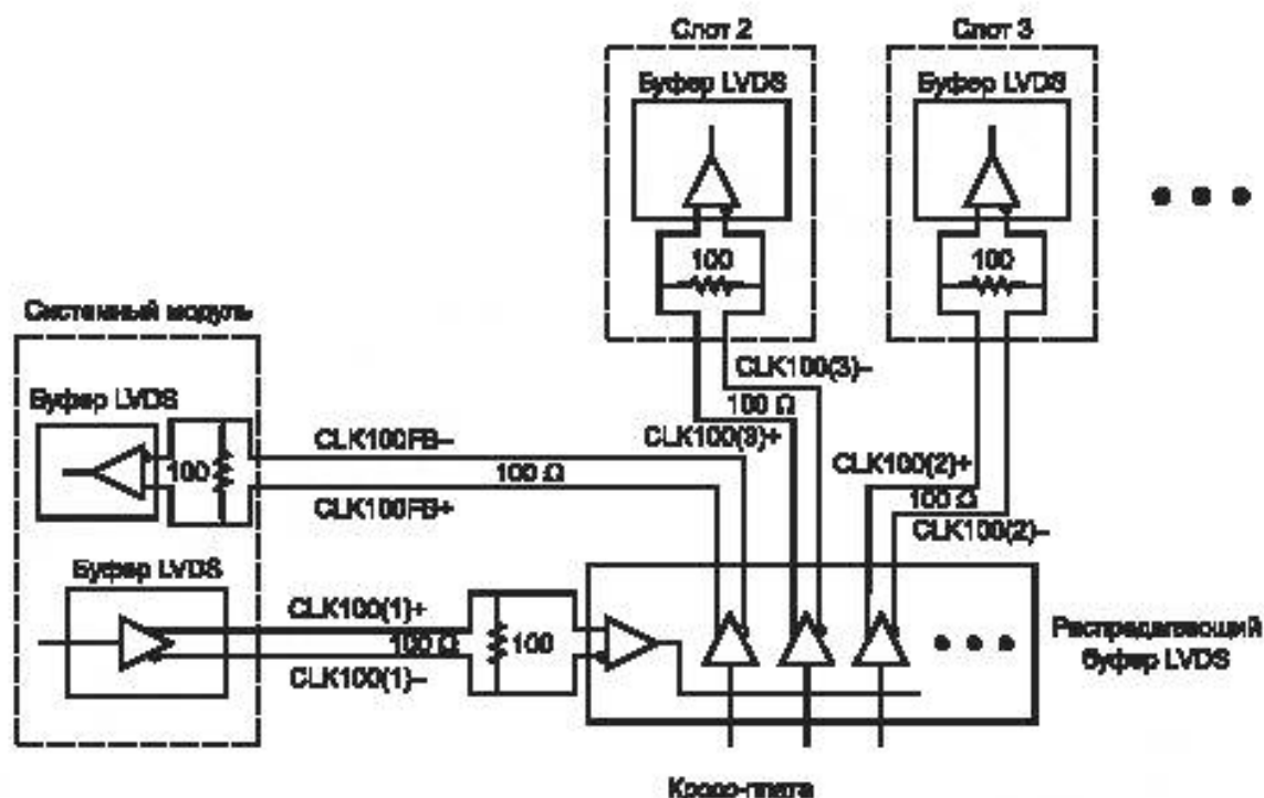
Рисунок 6.6 — Типичная реализация сигналов CLK100
