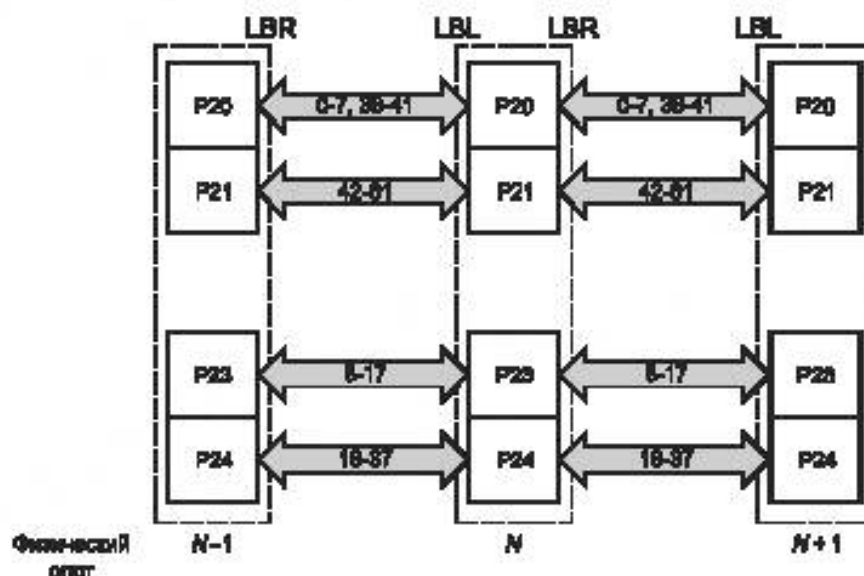
Рисунок 6.1 — Топология локальной шины кросс-платы AXIe
