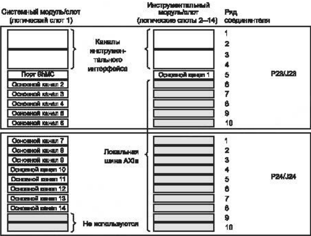
Рисунок 6.2 — Назначения канала основного интерфейса
