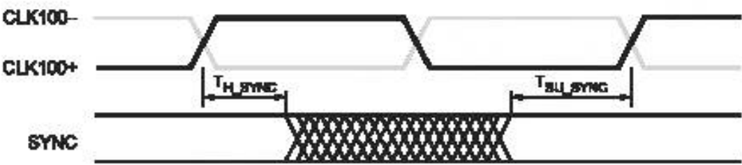
Рисунок 6.5 — Синхронный режим сигнала SYNC
