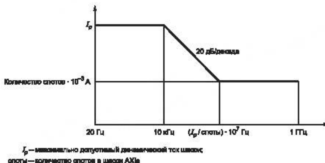
Рисунок 7.1 — Ток нагрузки шасси
