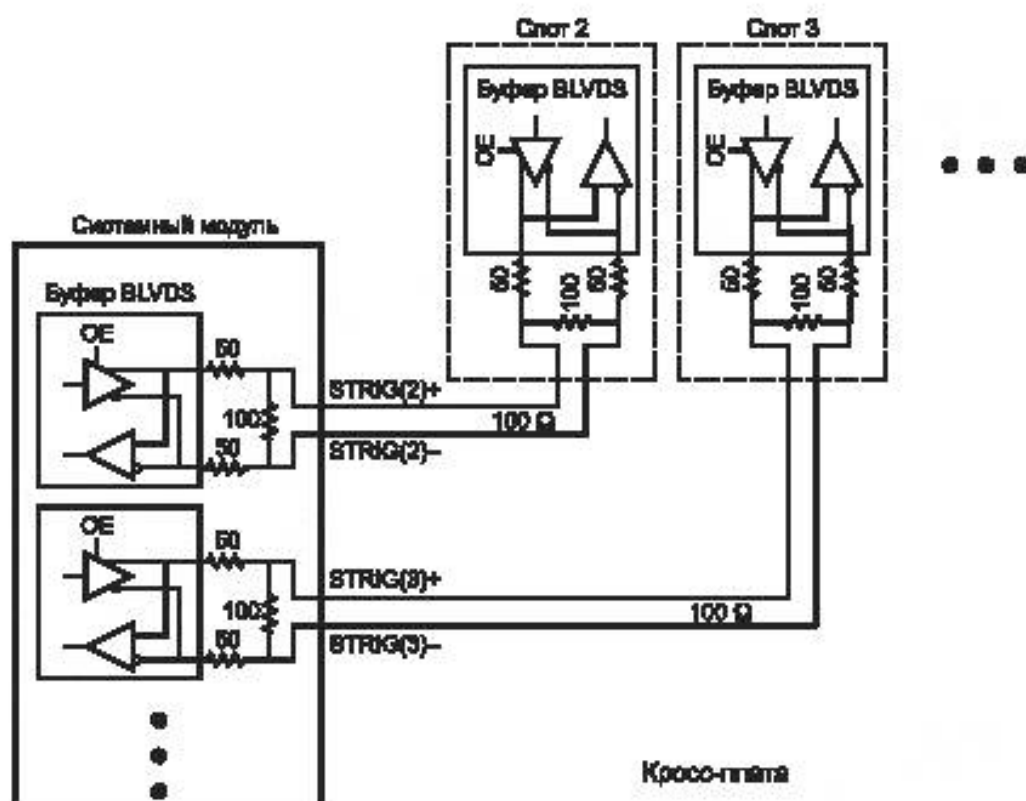
Рисунок 6.3 — Типичная реализация STRIG
