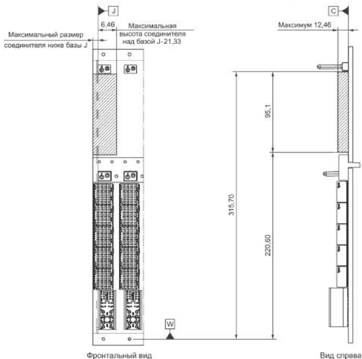
Рисунок 2.2 — Расположение соединителя зоны 3 кросс-платы AXIe-3.1
