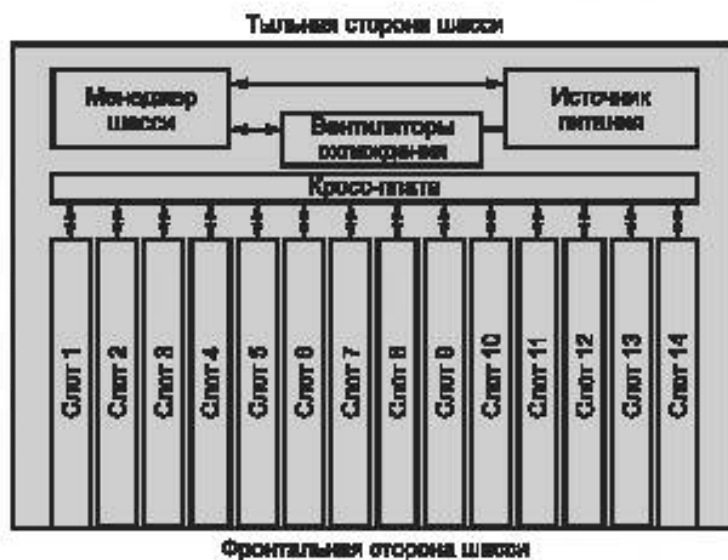
Рисунок 2 — Схема шасси AXIe
