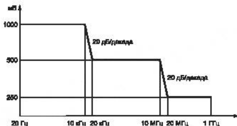
Рисунок 7.2 — Суммарная введенная помеха и пульсации напряжения питания
