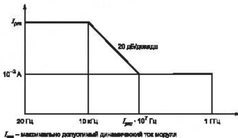
Рисунок 7.3 — Кондуктивные помехи модуля
