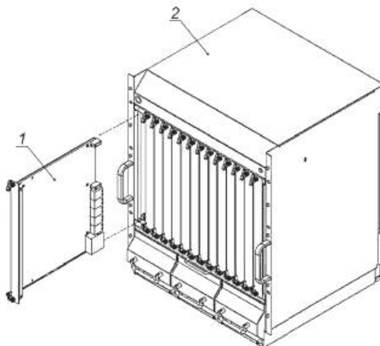
1 — модуль AXIe; 2 — шасси AXIe
