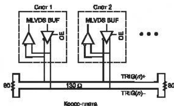
Рисунок 6.8 — Типичная реализация шины триггеров AXIe
