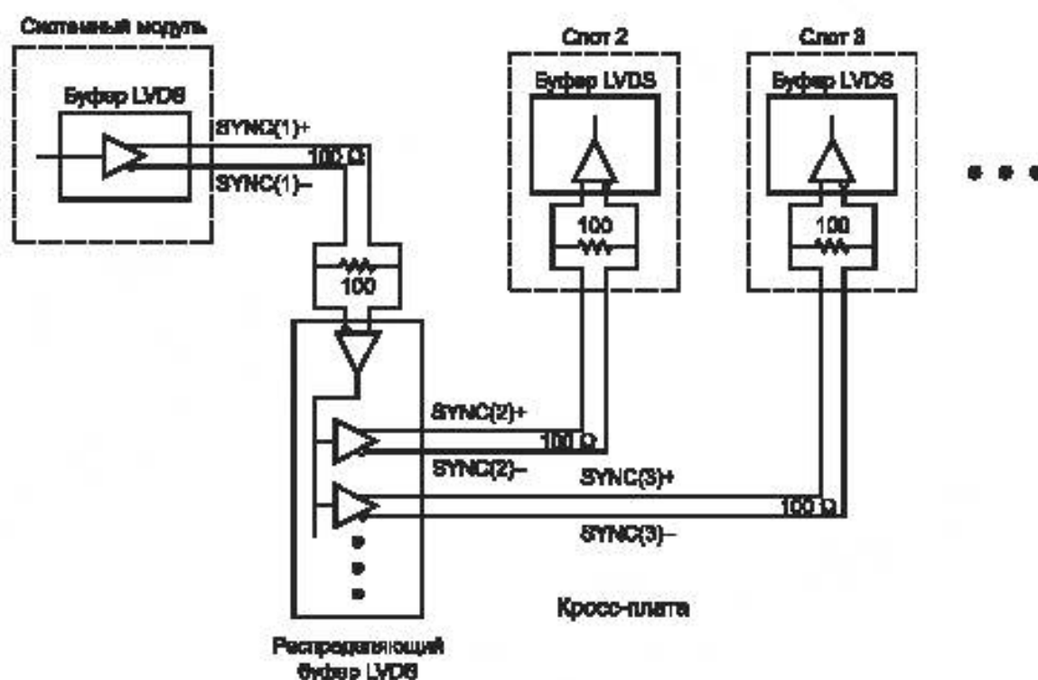
Рисунок 6.4 — Типичная реализация линий SYNC
