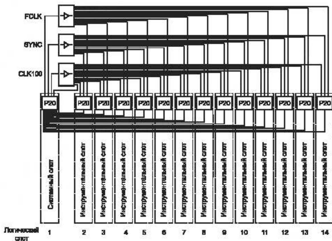
Рисунок 5 — Интерфейс синхронизации AXIe
