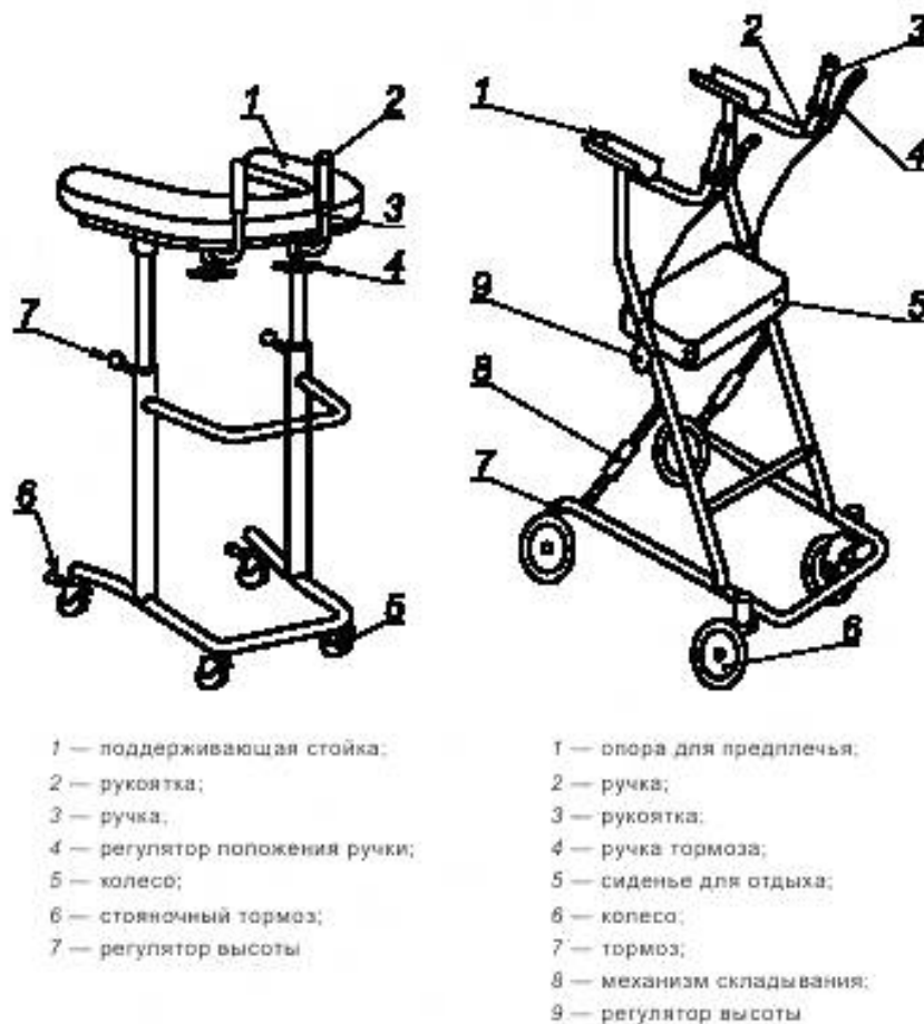
Рисунок 7 — Примеры стульчиков-ходунков на колесиках
