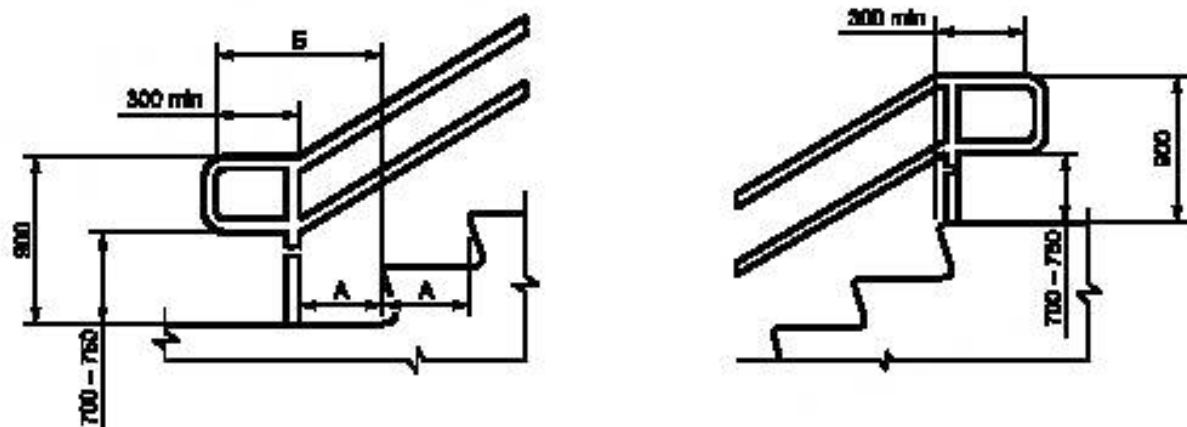
Рисунок 12 — Пример расположения поручней пандусов
