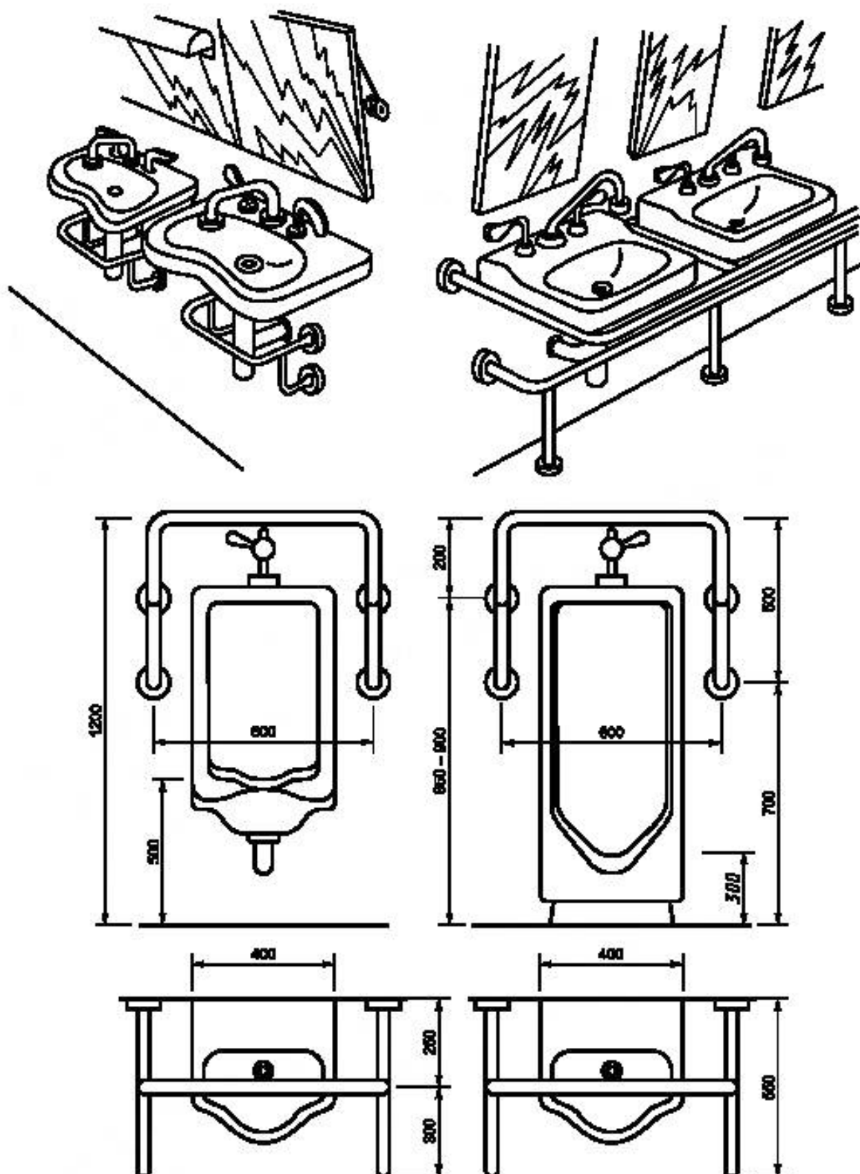
Рисунок 15 — Примеры оборудования поручнями ванных и душевых комнат
