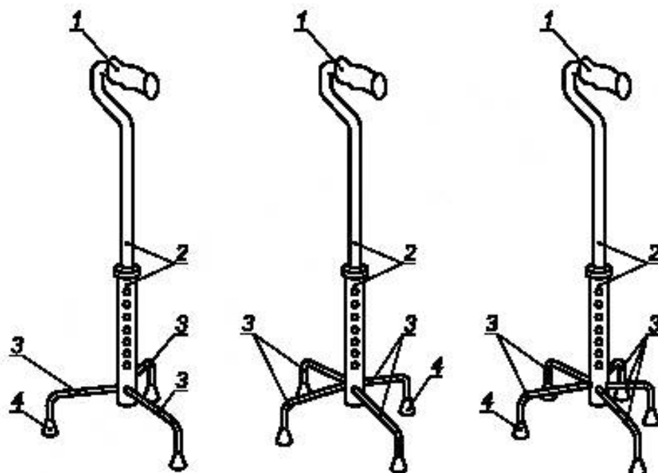
1 — ручка; 2 — стойка; 3 — ножка; 4 — наконечник
