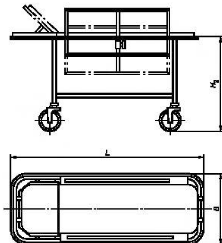
Рисунок 11 — Пример тележки для перевозки детей
