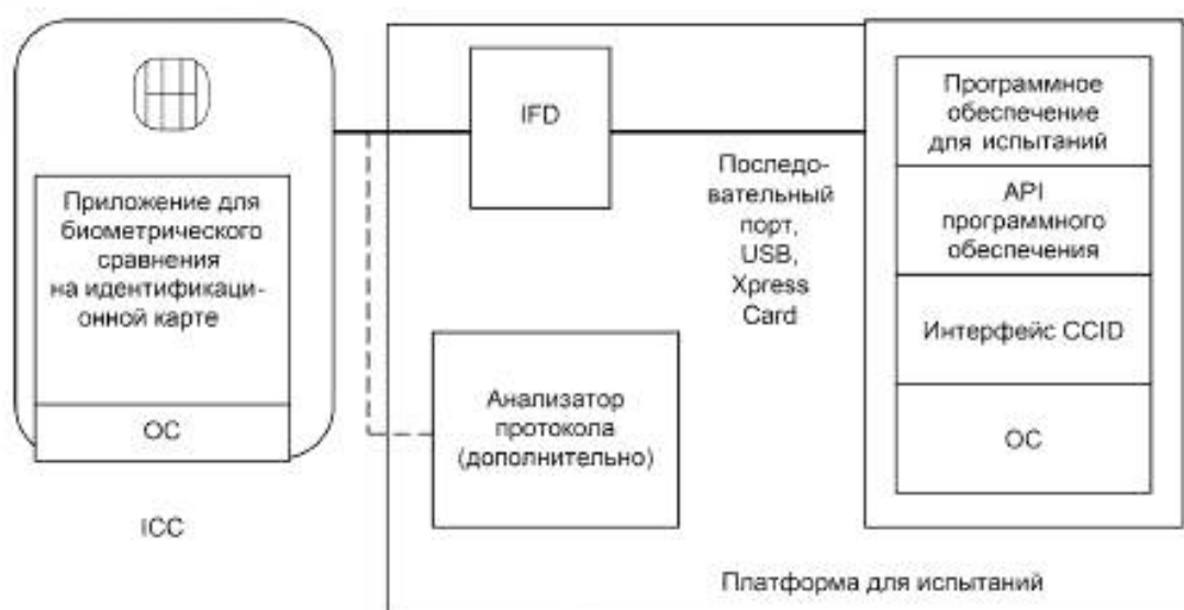
Рисунок В.1 — Обобщенная архитектура испытательной установки
