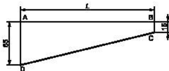
Рисунок 2 — Образец для испытаний типа 2 (клиновидный)
