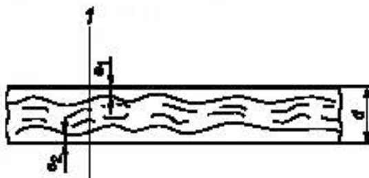
d — общая толщина; e_1 — толщина верхней обкладки; e_2 — толщина нижней обкладки; 1 — заданная точка измерения
