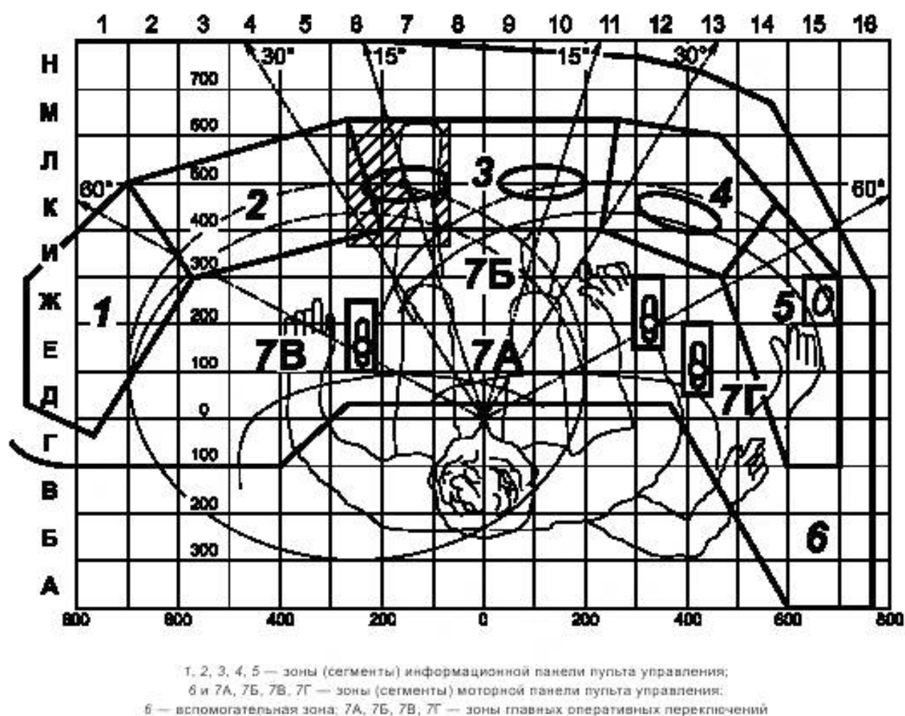
Рисунок 1 — Компонировка пульта управления
