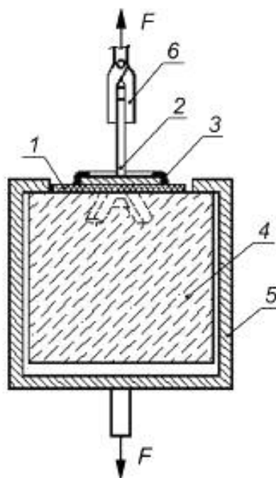
1 — фрагмент оболочки; 2 — антабка; 3 — сварной шов; 4 — бетонный куб; 5 — облойма; 6 — захват разрывной машины; F — усилие выдергивания
