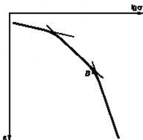
Рисунок Г.2 — Определение точки B при двух точках перелома графика
