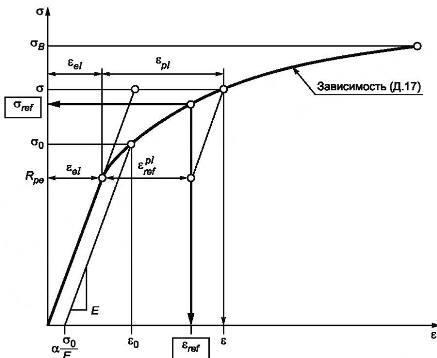
Рисунок Д.2 — Истинная диаграмма деформирования материала \sigma(\varepsilon)
