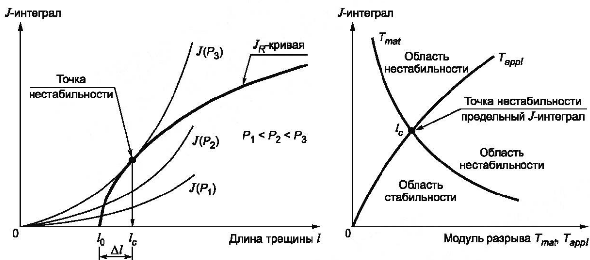
Рисунок Д.3 — Иллюстрация стабильного роста трещины на диаграммах J/J_R и J/T_{appl}
