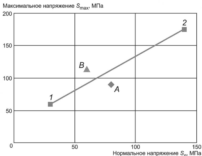
Рисунок Ж.1 — Линейная аппроксимация типичной ГРК
