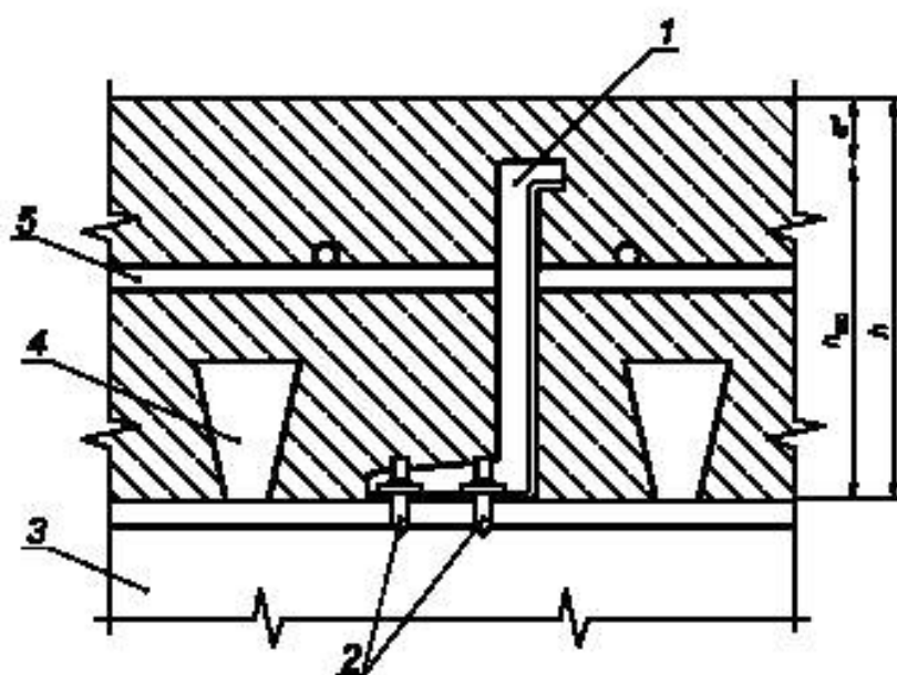
1 — уголкового упор; 2 — дюбель; 3 — балка; 4 — настил; 5 — плита
