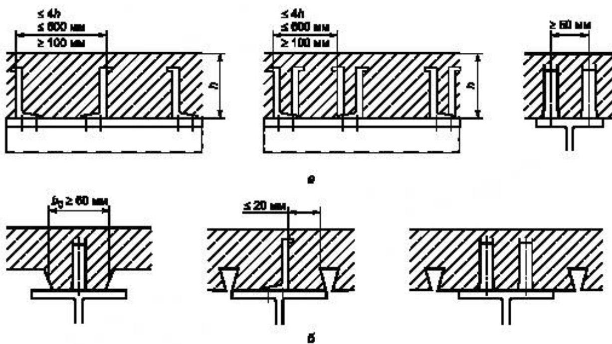
Рисунок 4 — Ориентация угловых упоров
