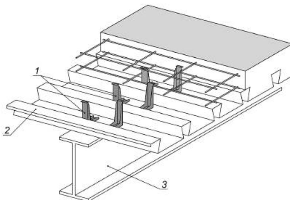
1 — уголкового упор; 2 — профилированный настил; 3 — балка
