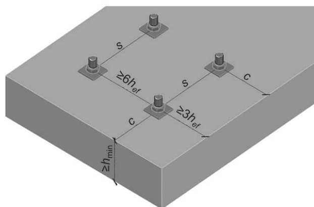
а) Принципиальная схема расположения анкеров на бетонном основании
