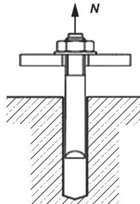
б) Разрушение по контакту с основанием
