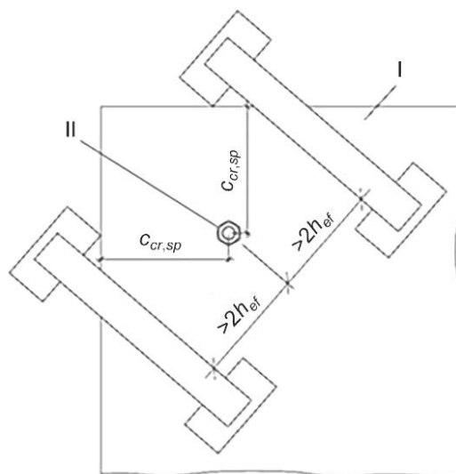
б) Пример оснастки для испытаний на растяжение анкеров, установленных в углу
