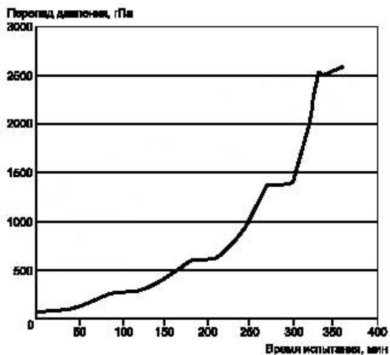
Рисунок В.2 — Типовая кривая загрязнения
