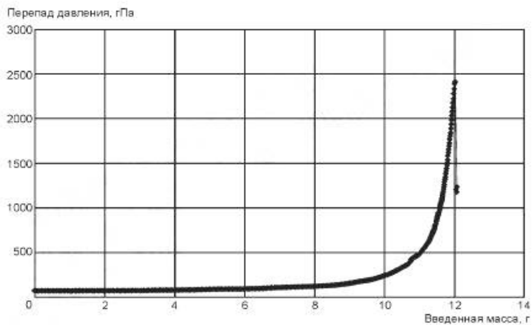
Рисунок В.4 — Типовая кривая разрушения
