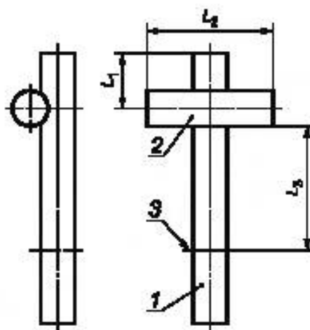
1, 2 — стержни; 3 — граница закрепления в захвате разрывной машины
