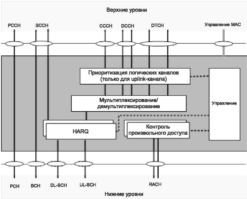
Рисунок 18 — Структура уровня MAC
