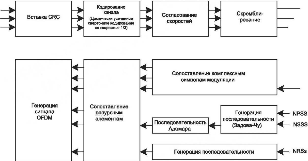
Рисунок 13 — Обработка физического downlink-канала
