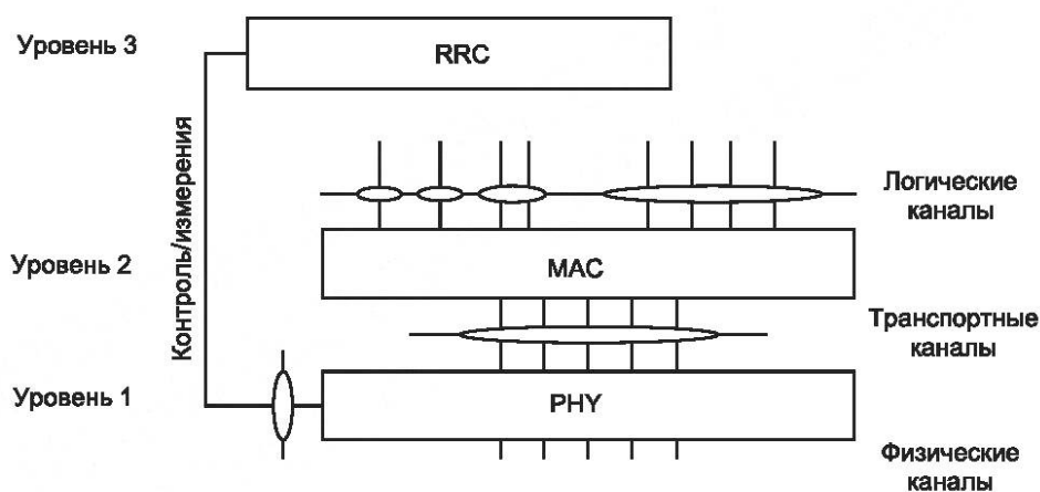
Рисунок 10 — Взаимосвязь уровней стека и каналов передачи данных
