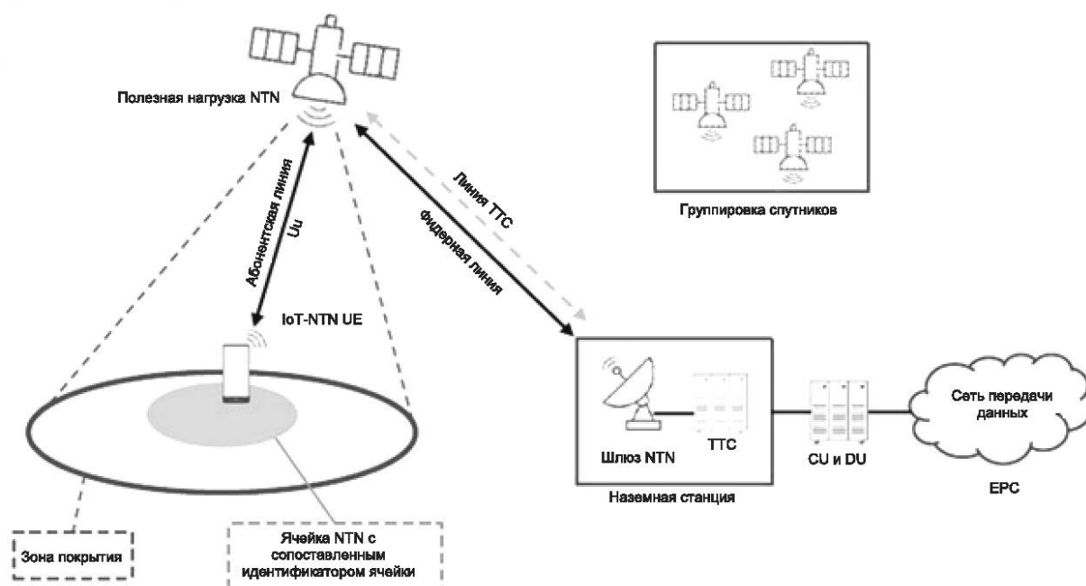
Рисунок 32 — Схема NTN-связи
