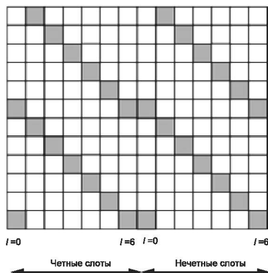
Рисунок 16 — Распределение NPRS ( operationModeInfoNPRS установлен на режим работы Standalone или Guard-band, nprsBitmap сконфигурирован)
