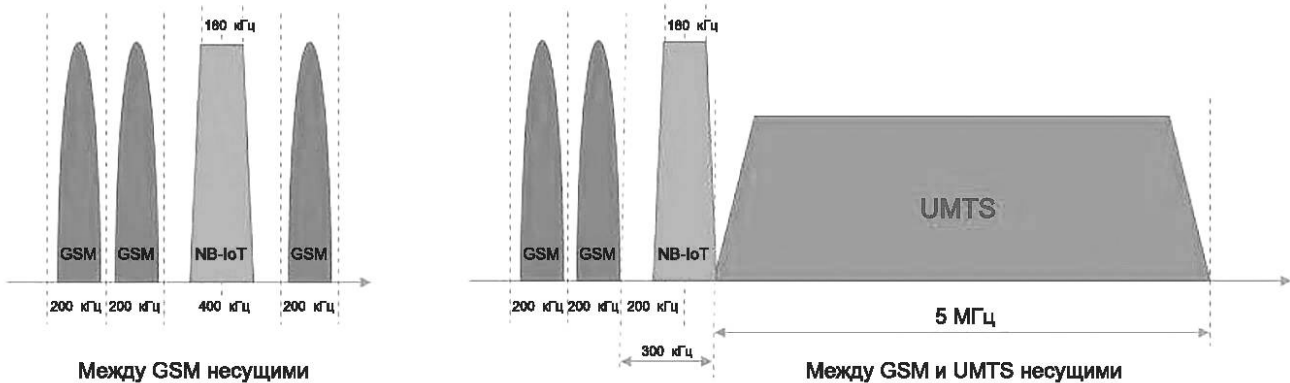
Рисунок 1 — Варианты размещения канала NB-IoT в режиме Standalone
