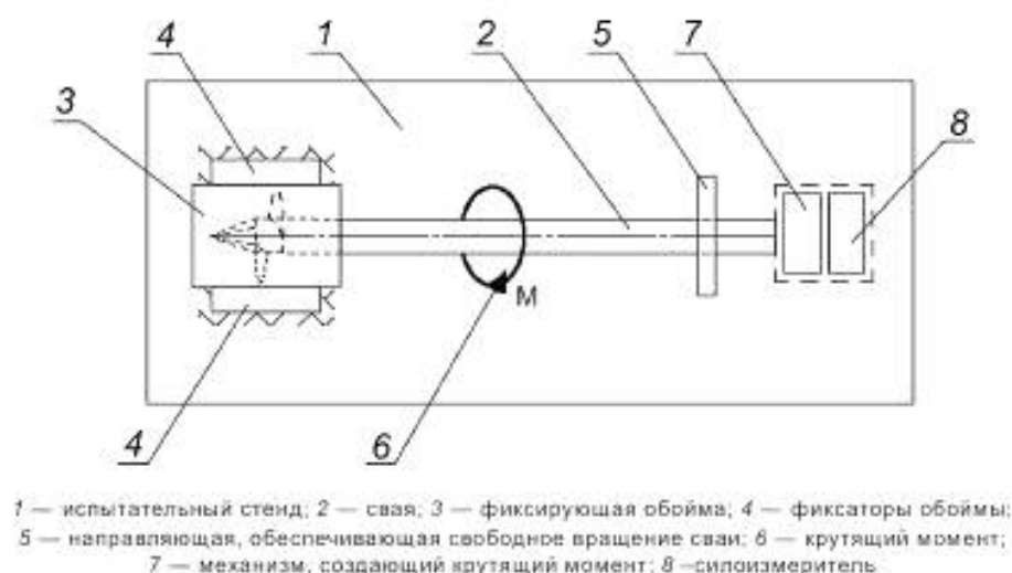
Рисунок Б.2 — Схема испытания сваи крутящим моментом
