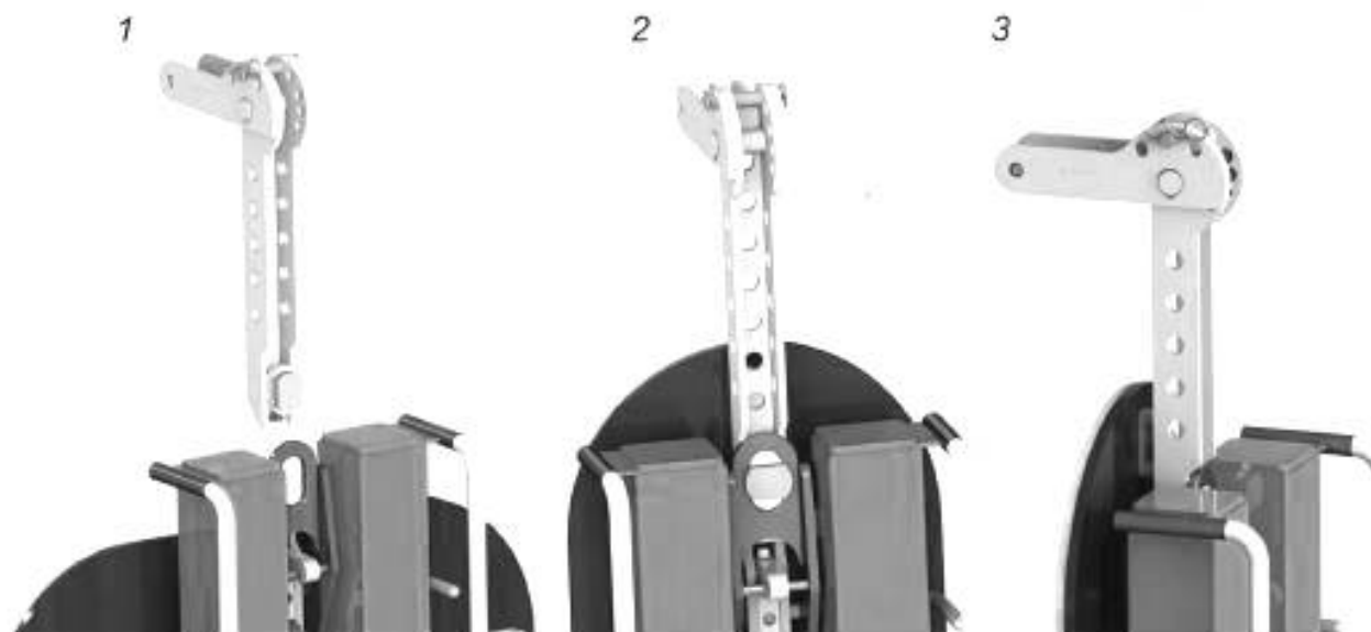
1 — установка кронштейна; 2, 3 — установленный кронштейн развесовки
