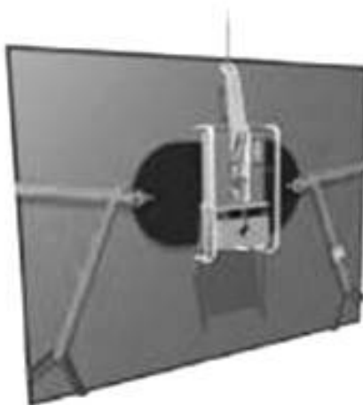
Рисунок 10 — Страховочное устройство в комплекте с вакуумным захватом для стекол
