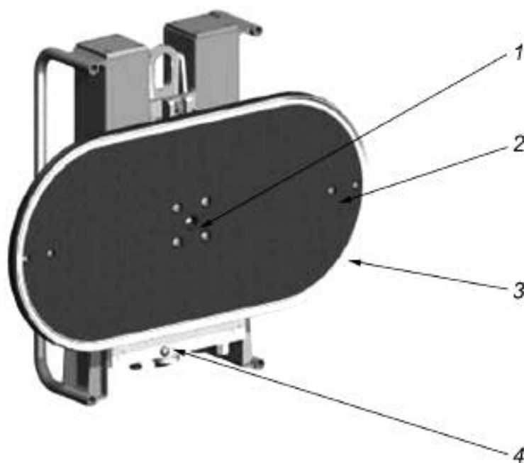
1 — вакуум-фильтр; 2 — фрикцион; 3 — уплотнительный профиль; 4 — фильтр продувки
