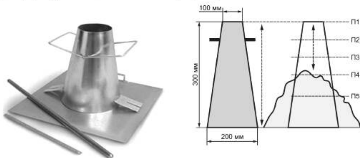
Рисунок 1 — Общий вид прибора и схема определения подвижности бетонной смеси по осадке конуса, отформованного из бетонной смеси марок П1, П2, П3, П4, П5
