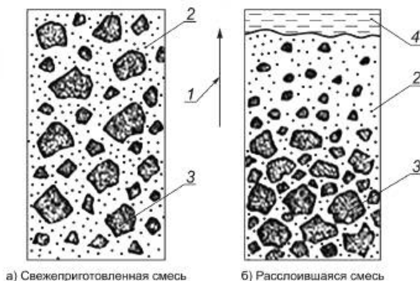
Рисунок 8 — Расслоение бетонной смеси при длительных вибрационных воздействиях
