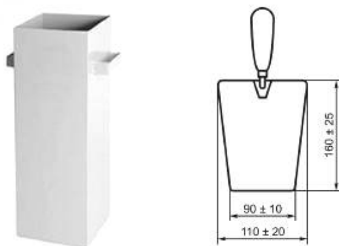
Рисунок 4 — Форма для определения степени уплотняемости бетонной смеси и кельма
