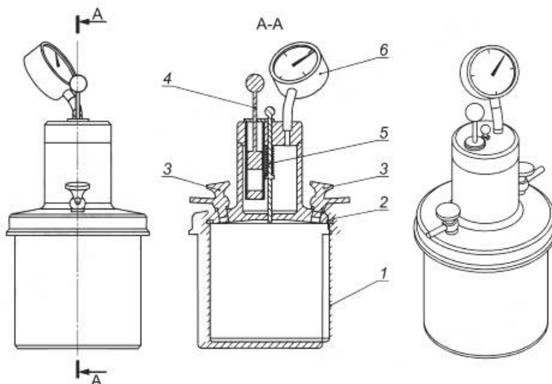
1 — чаша; 2 — крышка; 3 — зажим; 4 — ручной насос; 5 — выпускной клапан; 6 — манометр
