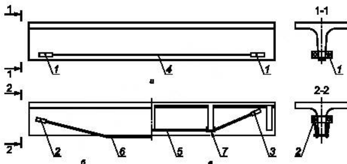
1—3 — анкерные узлы различной конструкции; 4 — прямолинейные и 5 — полигональные шпренгели (напрягаемые затяжки); 6, 7 — оттяжки (огibaющие устройства) различной конструкции
