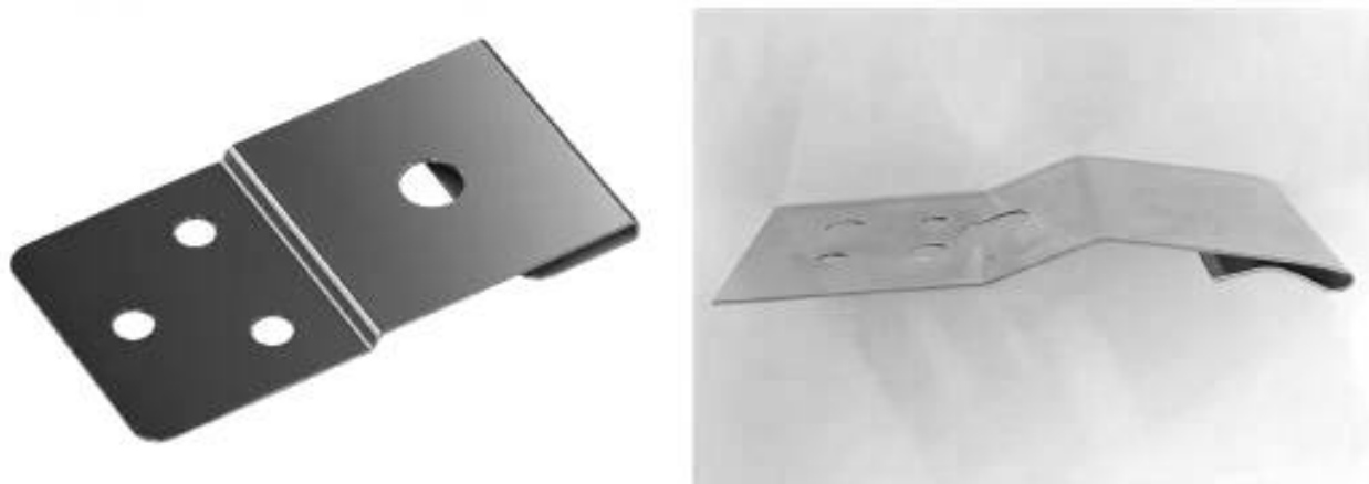
Рисунок 4 — Кляммер для лежачего фальца, примеры
