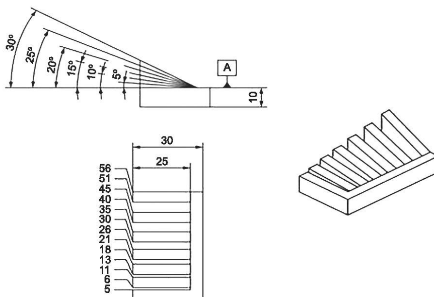
Рисунок 10 — Общий вид крупного элемента со скошенными плоскостями
