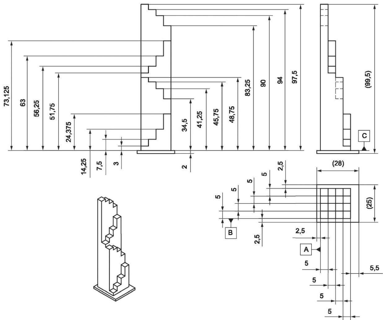
Рисунок 4 – Общий вид среднего ступенчатого образца для испытаний
