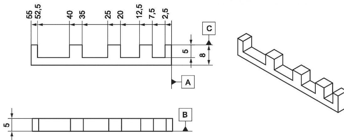
Рисунок 1 — Общий вид линейных образцов
