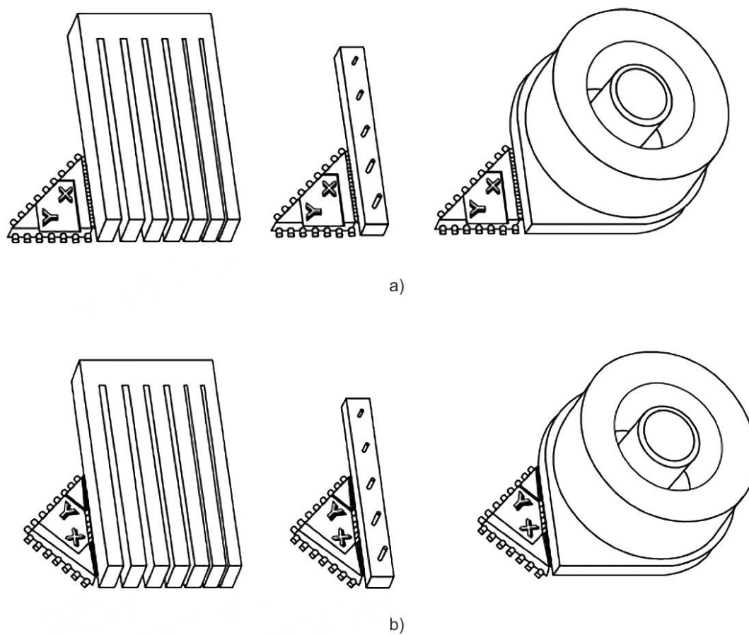
Рисунок 14 — ХУ-ярлыки, присоединенные для построения под углом 0°, 90° [вариант а)] и под углом 45° [вариант б)]
