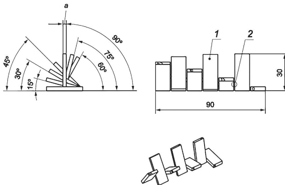
1 — пластинка размерами 12,0 × 30,0 × 3,0 мм; 2 — соединительная подпорка (одна из шести); a — толщина пластинки
