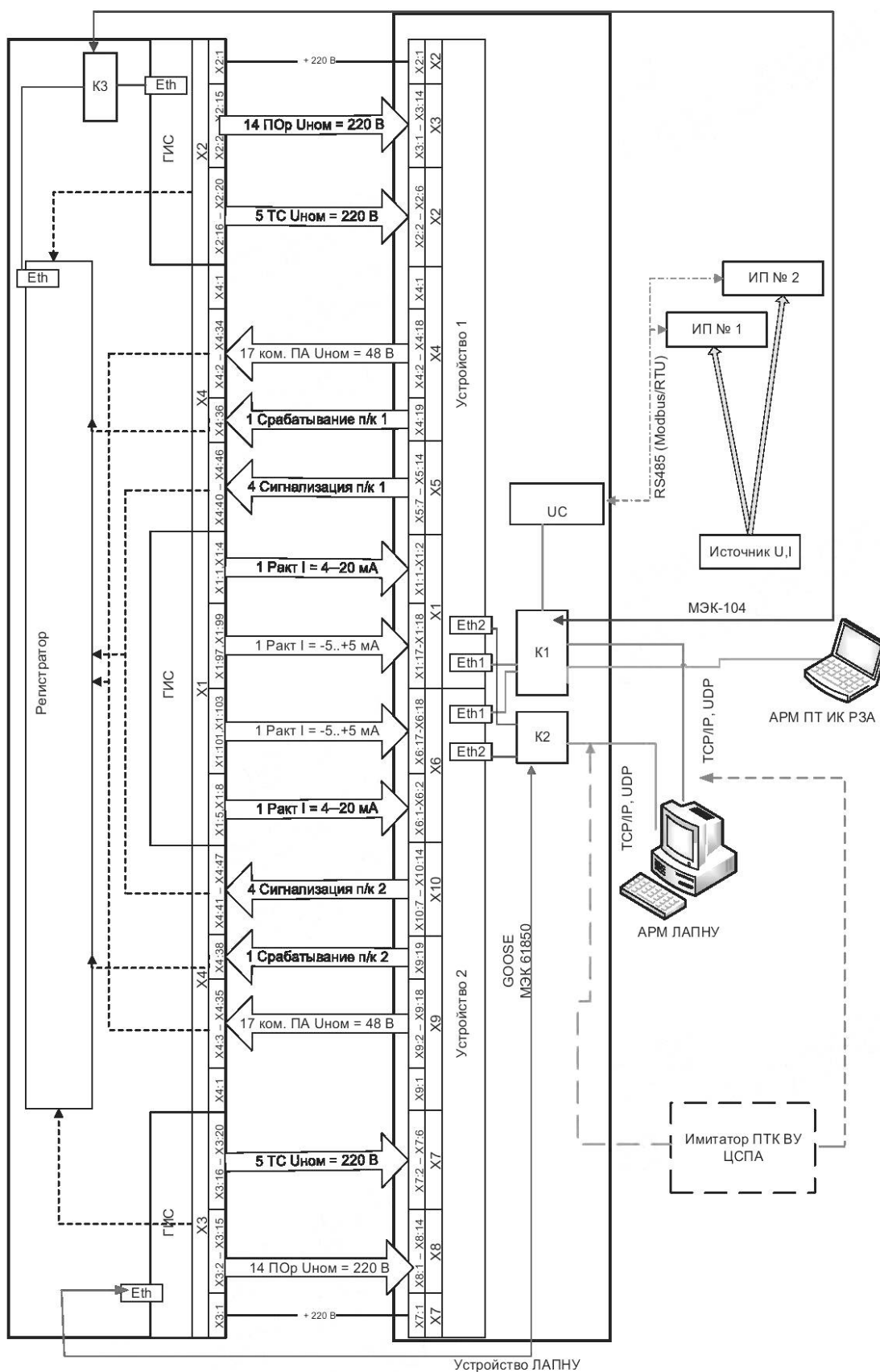
Рисунок Б.2 — Пример тестовой схемы для испытаний устройств ЛАПНУ
