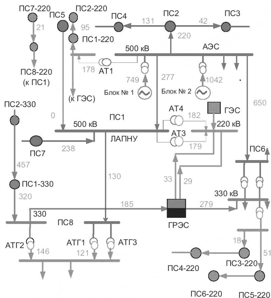
Рисунок Б.1 — Поясняющая схема контролируемого энергорайона
