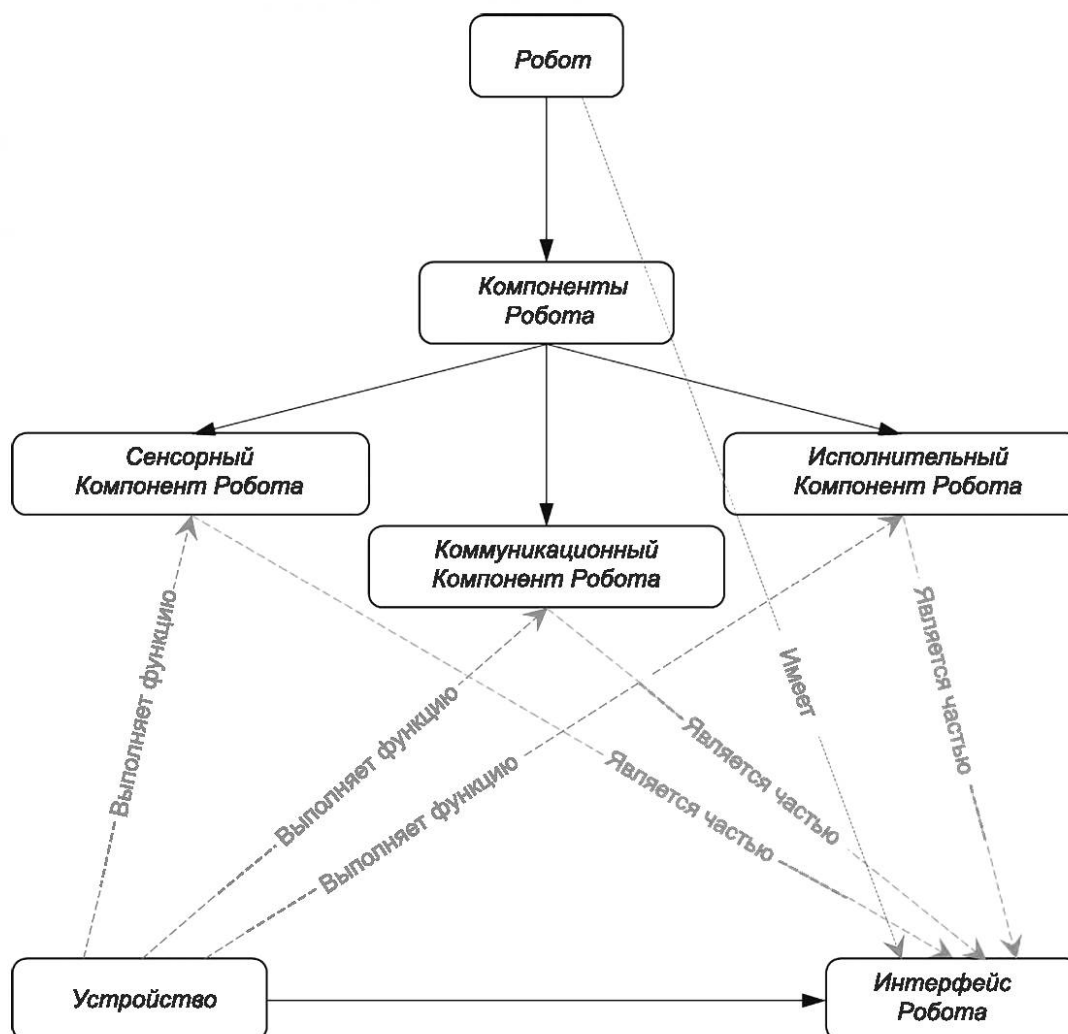
Рисунок 3 — Таксономия понятия Интерфейс Робота
