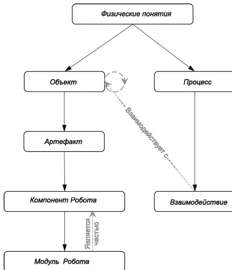
Рисунок 4 — Таксономия понятия Модуль Робота
