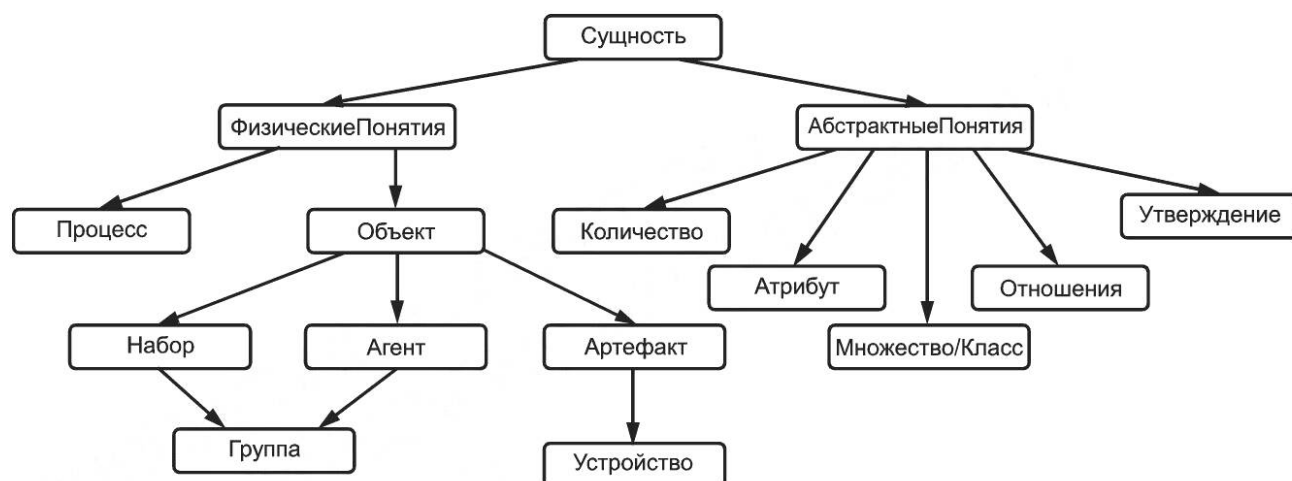
Рисунок 1 — Базовая таксономия SUMO
