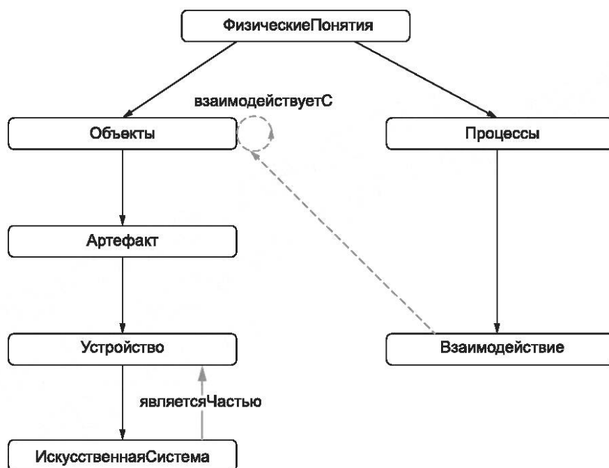
Рисунок 3 — Таксономия понятий Искусственная Система и Взаимодействие по CORAX
