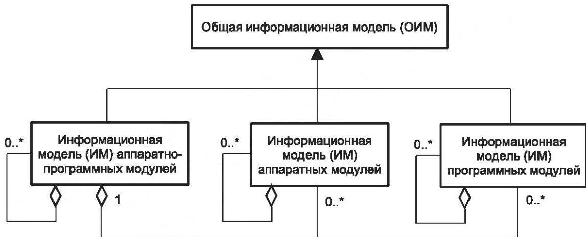
Рисунок 4.1 — Взаимосвязи между информационными моделями модулей
