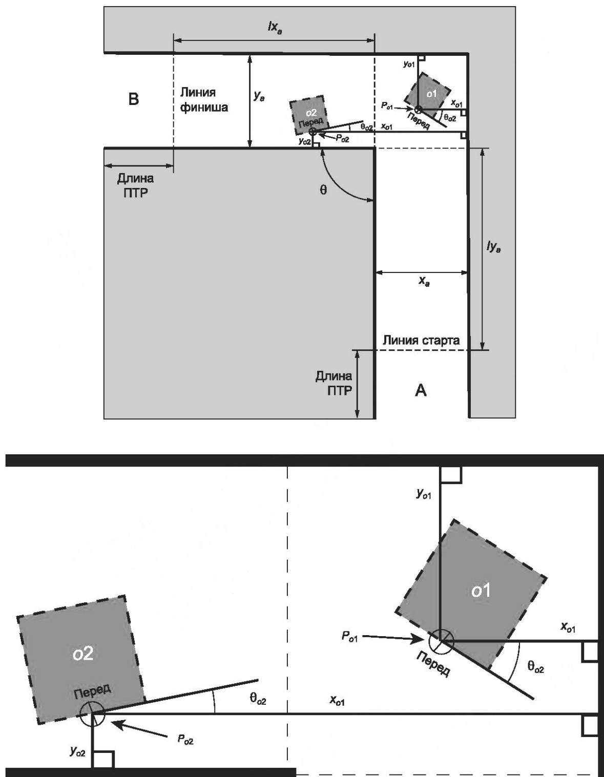
Рисунок 16 — Сверху: оборудование прямого прохода в заданной области с двумя препятствиями ( o1 и o2 ). Снизу: подробное изображение площади препятствий в основании и параметров, определяющих их позиции, ориентации и начала координат
