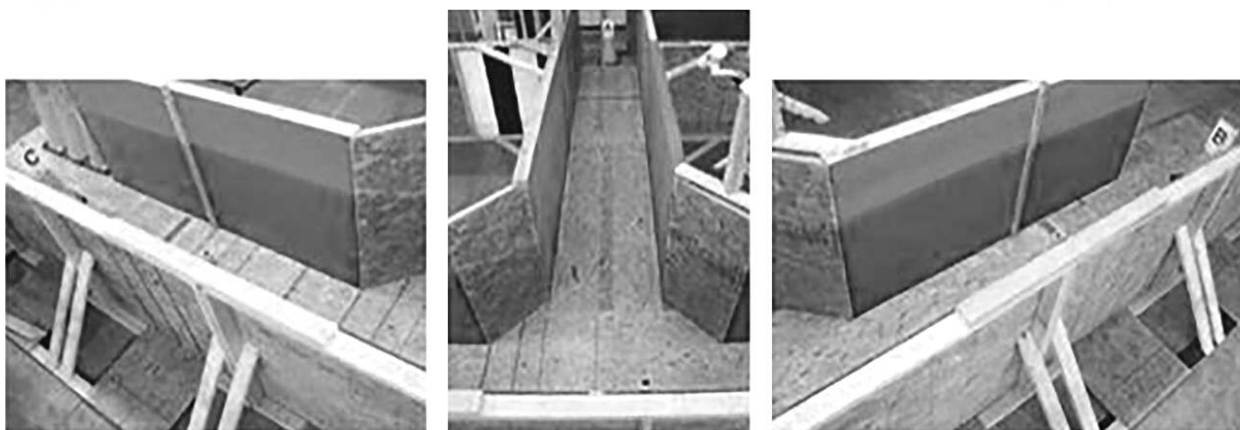
Рисунок 9 — Пример оборудования Т-образного перекрестка с физическими ограждениями
