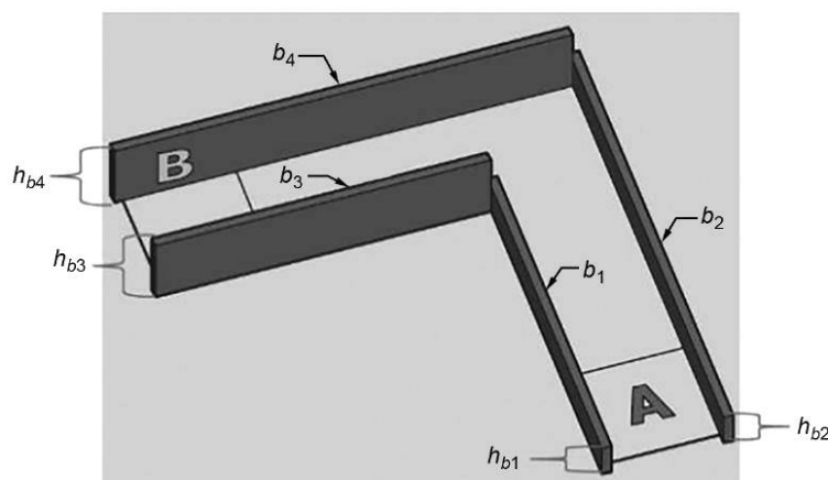
Рисунок 12 — Угловое пересечение, образованное оборудованием заданной зоны с четырьмя разными значениями высоты сегментов
