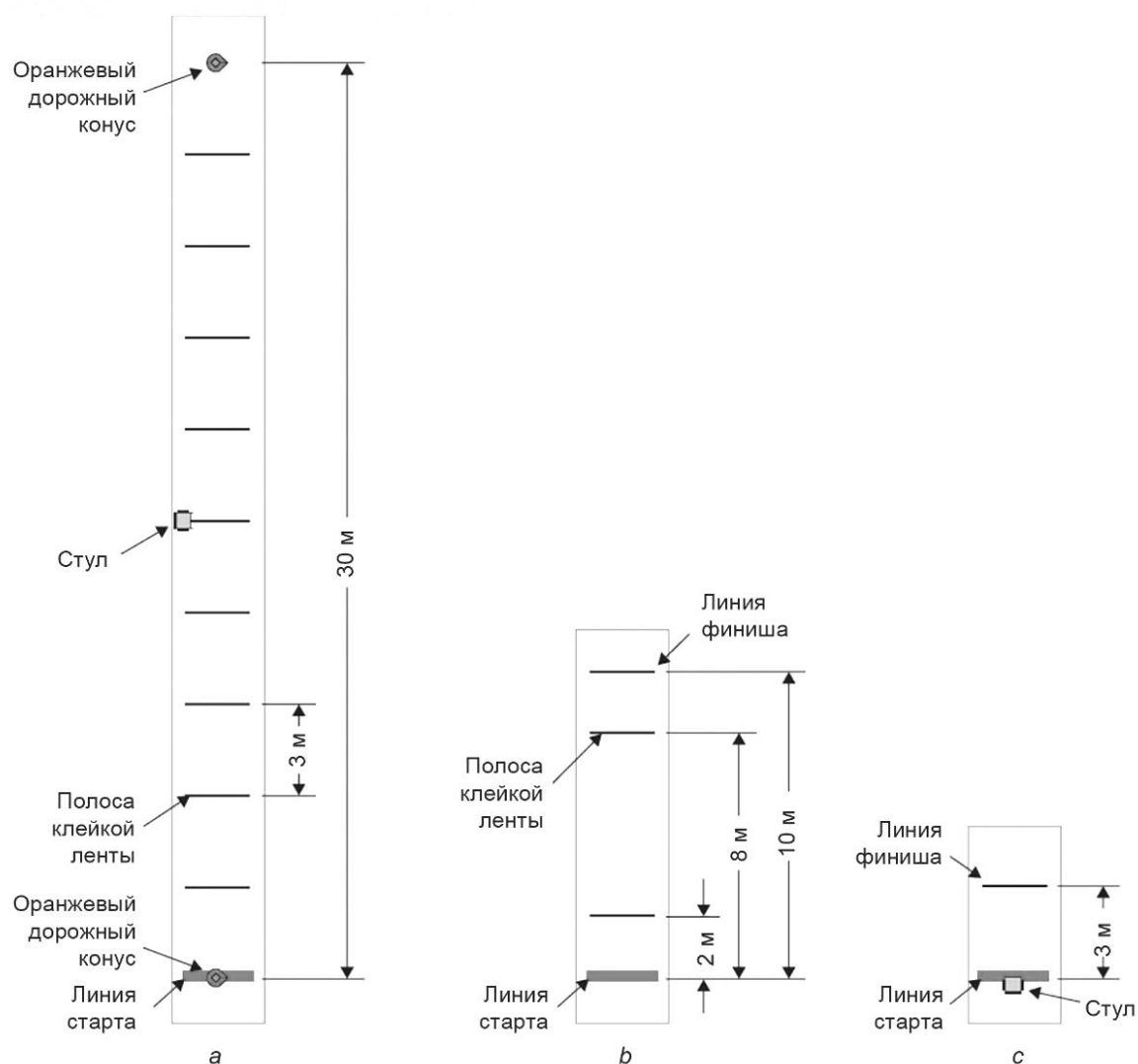
а — испытание 6МХ; б — испытание 10МХ; в — испытание ВИ
