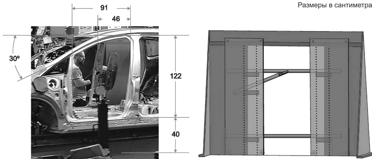
a — пример реального проема под дверь автомобиля
