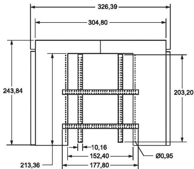
б – вид спереди
