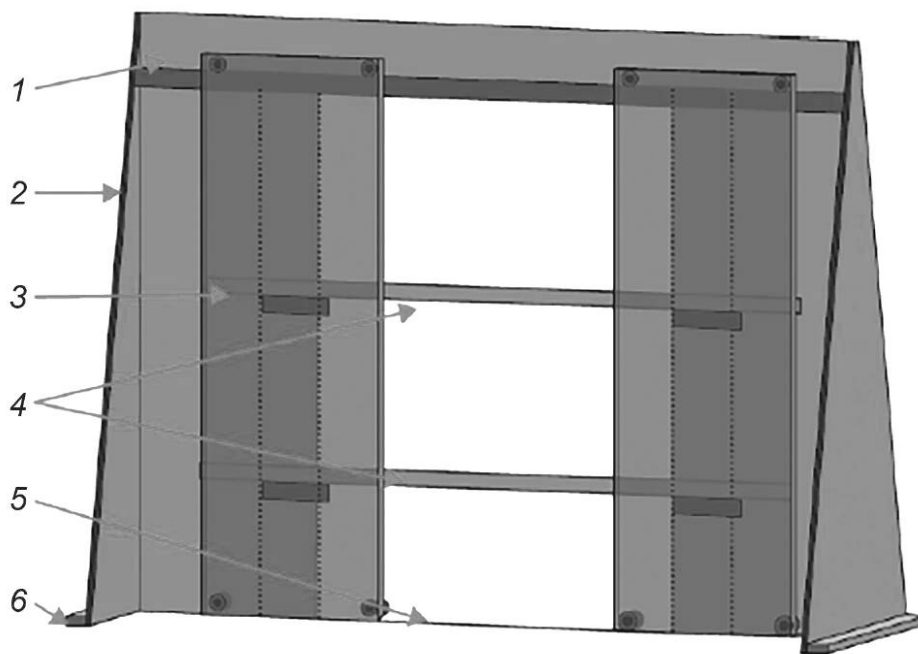
а — общий вид испытательного оборудования
