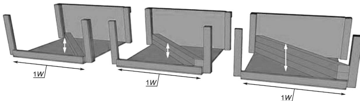
Рисунок 6 — Вид испытательного стенда с брусом разной высоты
