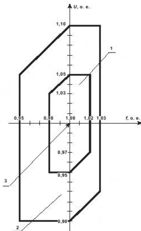
Рисунок 12 — Предельные значения напряжения и частоты для двигателей
