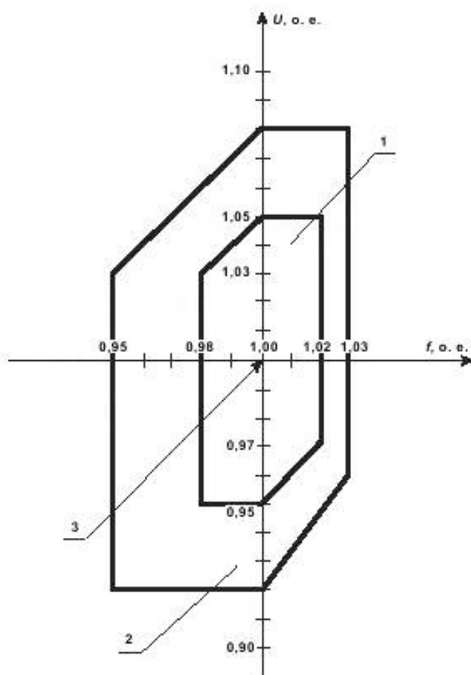
Рисунок 11 — Предельные значения напряжения и частоты для генераторов
