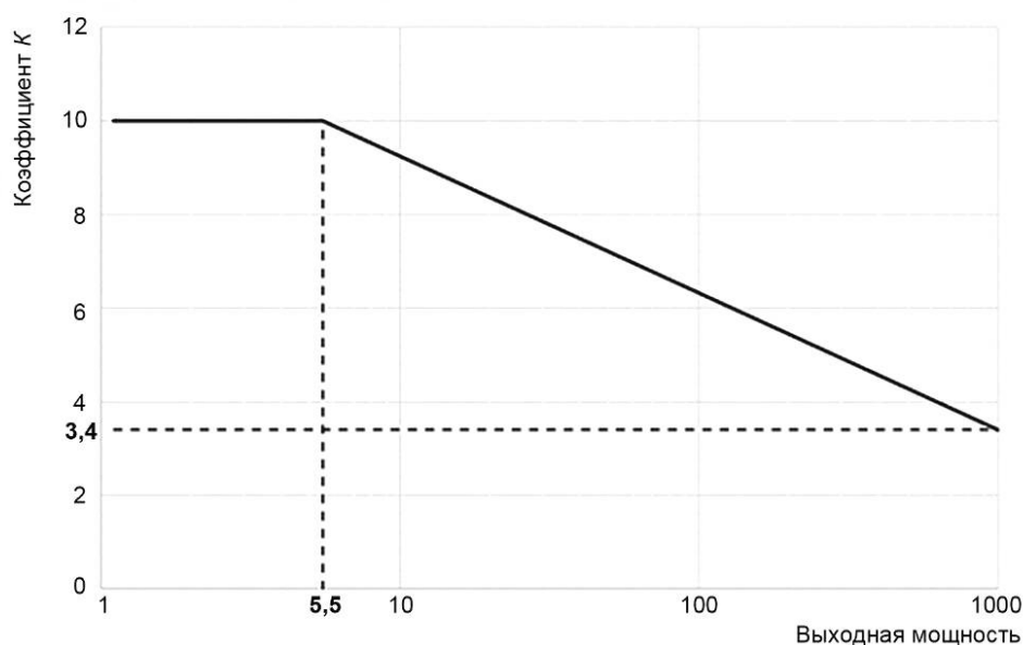
Рисунок 13 — Коэффициент K для определения R_{PE,M}
