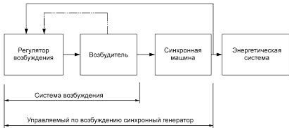
Рисунок 1 — Структура управляемого по возбуждению синхронного генератора
