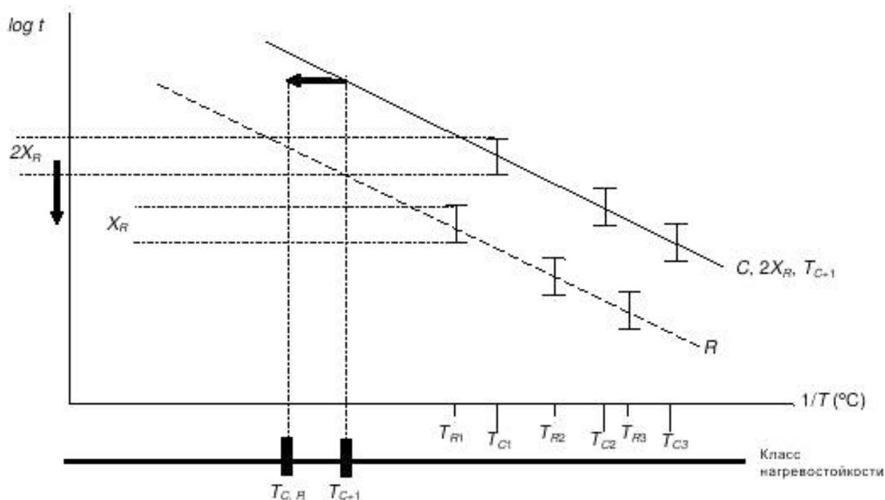
Рисунок 4 — Испытываемая система, аттестованная для другого срока эксплуатации и другого класса нагревостойкости по сравнению с эталонной
