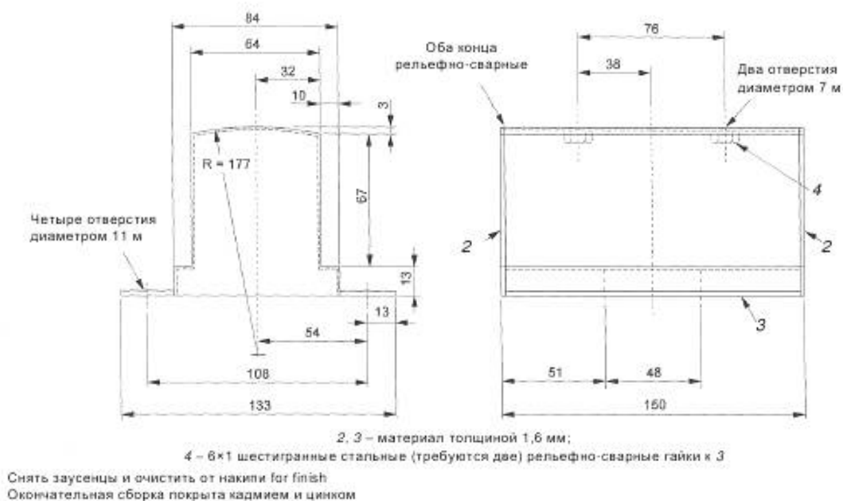
Рисунок В.7 — Производственный чертеж модели полюсного сердечника для измерения намотанной обмотки на испытательной арматуре
