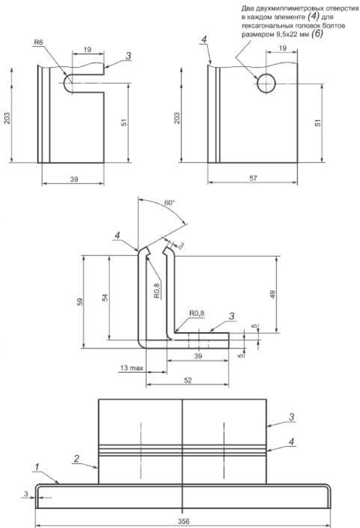
Рисунок А.2 — Типичный монтаж паза
