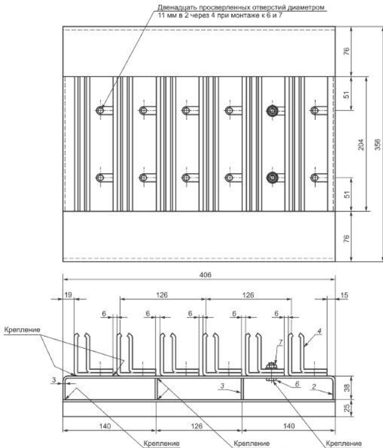
Рисунок А.1 — Типичный монтаж лаза
