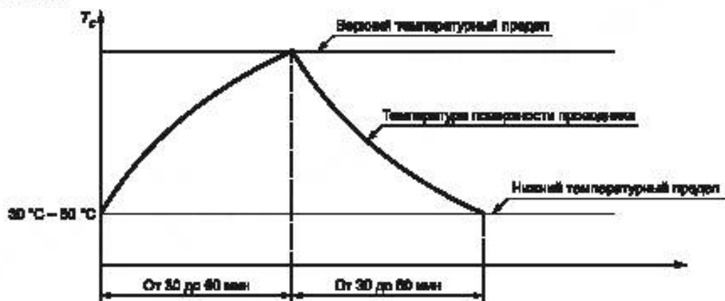
Рисунок 2 — График цикличности нагрева и охлаждения
