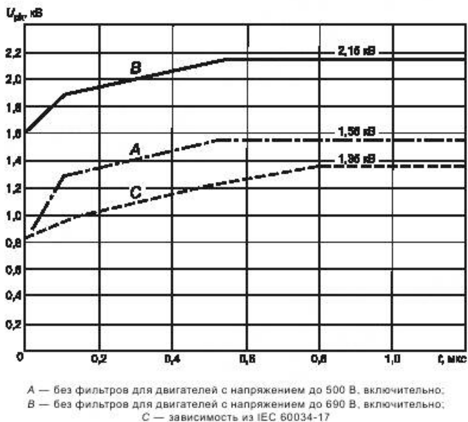
Рисунок А.2 — Граничные кривые импульсного напряжения U_{pk} , приложенного между двумя фазными зажимами двигателя в функции времени нарастания импульса t ,
