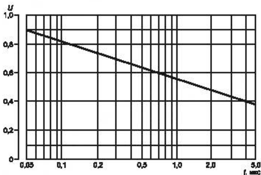
Рисунок 9 — Худший случай распределения напряжений в межвитковой изоляции разнообразных вспыхивающих обмоток статора в функции времени нарастания импульса
