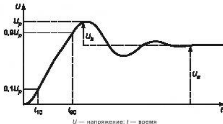
Рисунок 1 — Параметры импульса напряжения
