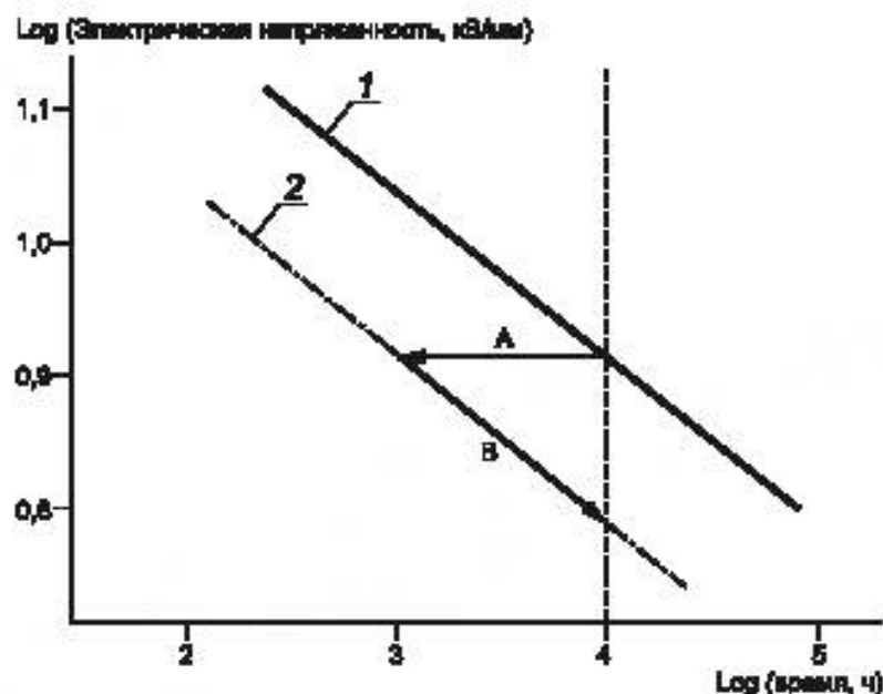
Рисунок 7 — Пример срока службы корпусной системы изоляции типа II
