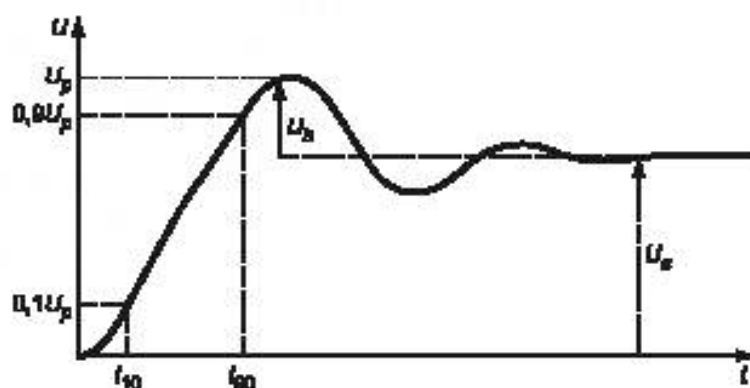
Рисунок 1 — Параметры импульса напряжения
