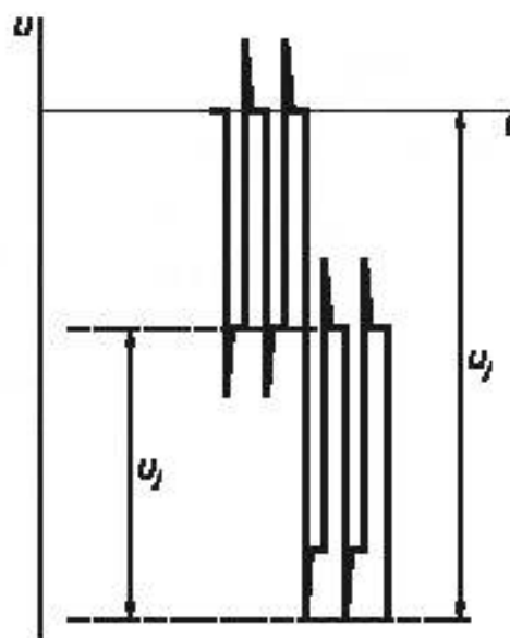
Рисунок 3 — Возможный скачок напряжения U_1 на зажимах машины, связанный с типом преобразователя
