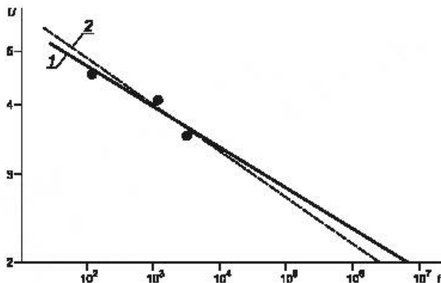
1 — срок службы межвитковой изоляции; 2 — срок службы корпусной изоляции; t — время до пробоя; U = U_{испыт}/U_{ном} — для витковой изоляции; U = U_{испыт}/U_{ном} — для корпусной изоляции
