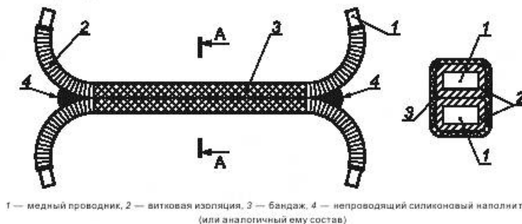
Рисунок 8 — Пример конструкции испытываемого образца межвитковой изоляции обмотки из прямоугольного провода
