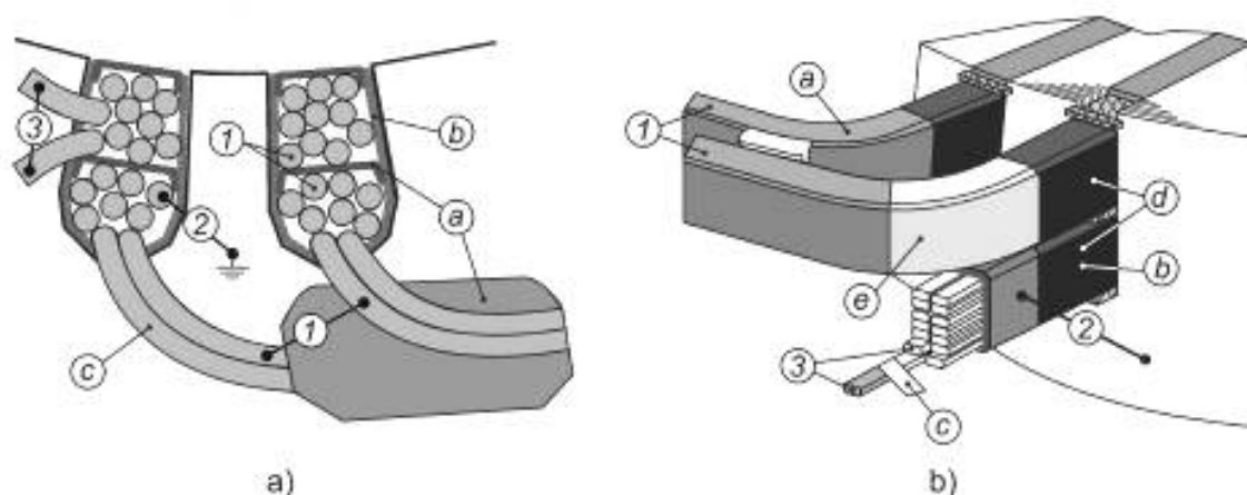
а — фазная изоляция (межспойная); б — изоляция на землю; с — витковая изоляция; d — система защиты от короны в пазу; e — система выравнивания напряженности электрического поля; 1 — межфазная изоляция; 2 — изоляция «фаза—земля»; 3 — межвитковая изоляция
