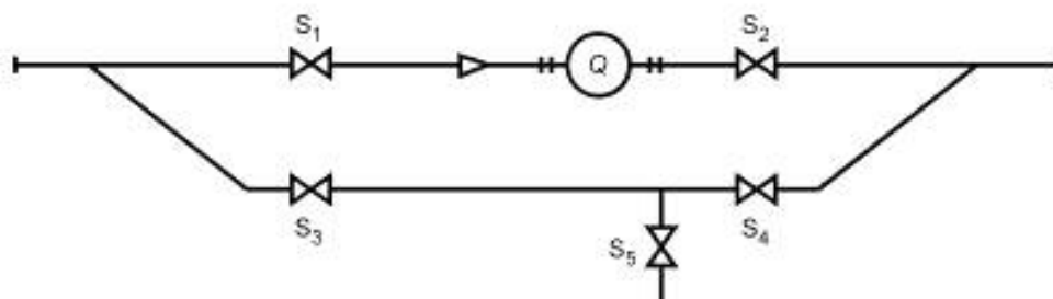
Рисунок 5 — Установка расходомера с обходным каналом
