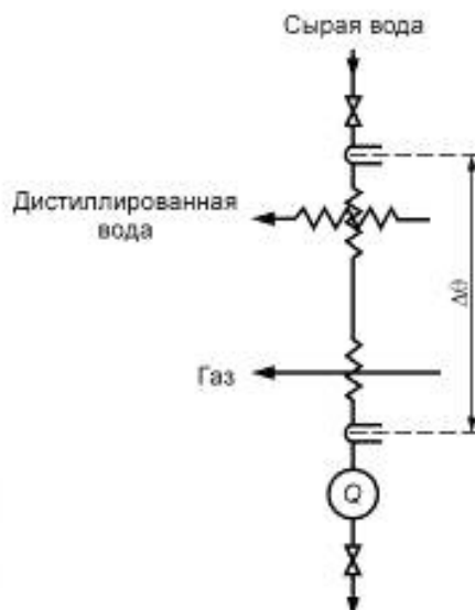
Рисунок 4 — Последовательное соединение охладителей, два хладагента
