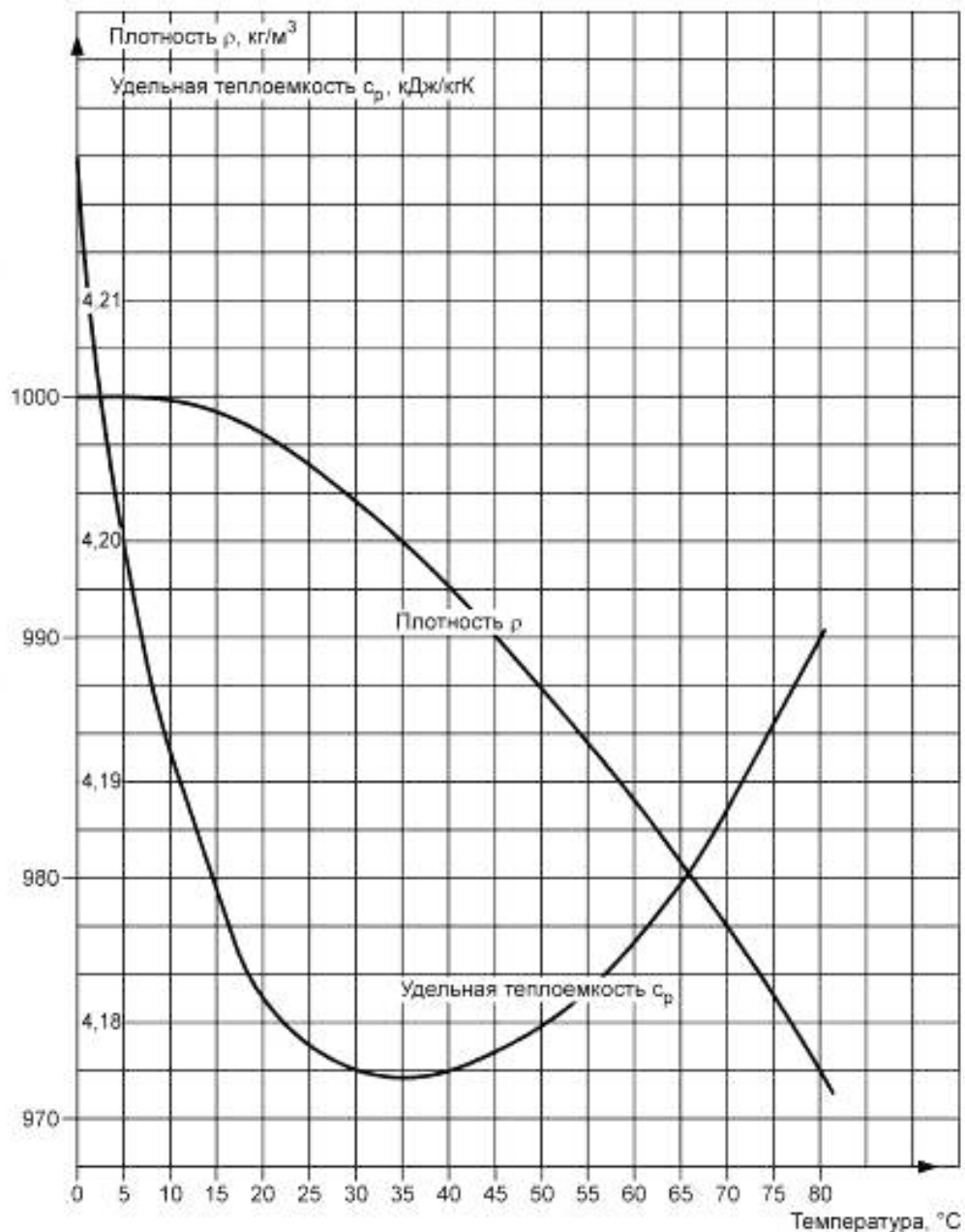
Рисунок 7 — Характеристики дистиллированной воды в функции температуры
