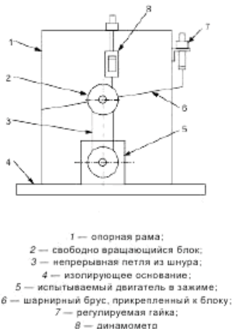
Рисунок В.4 — Метод измерения опрокидывающего момента при помощи шнура и динамометра
