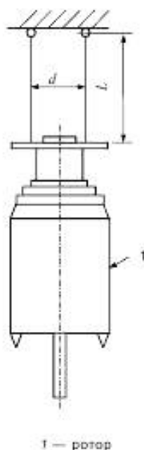
Рисунок А.1 — Метод измерения при помощи двух шнуров
