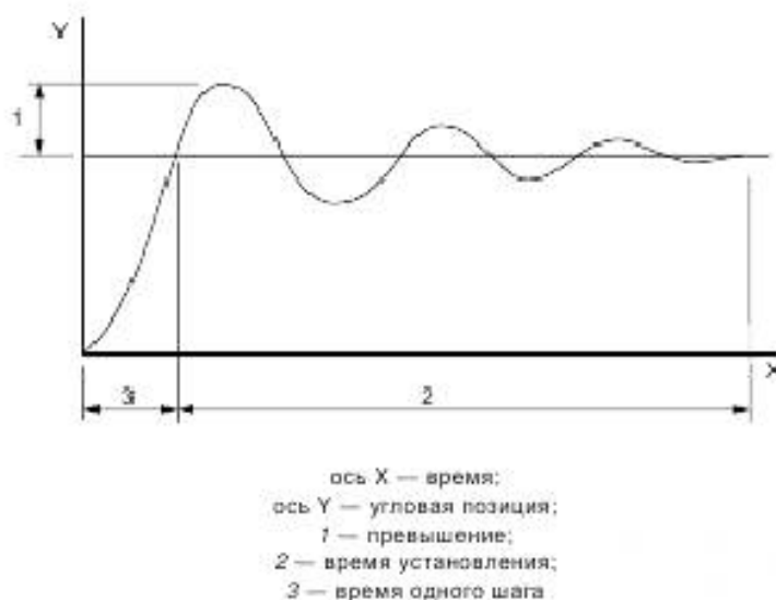
Рисунок 1 — Наибольшее значение и время установления
