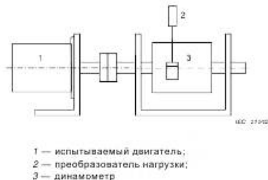
Рисунок В.3 — Испытательный стенд для измерения опрокидывающего момента при помощи динамометра
